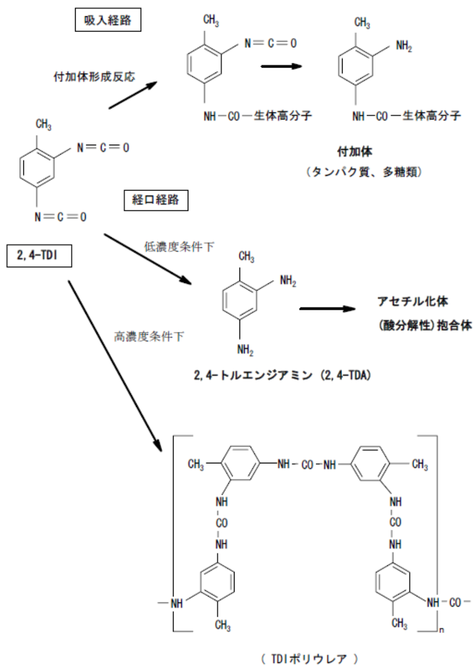
図 1-1 2,4-TDI の動物における主な代謝経路 (NITE, 2008a) (4 位のイソシアナート基が生体内高分子と結合した場合を示す。 2 位のイソシアナート基も生体高分子に結合する可能性がある。)
