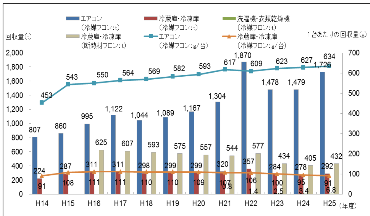
図表 4 製造業者等による冷媒フロン・断熱材フロンの回収量の推移
