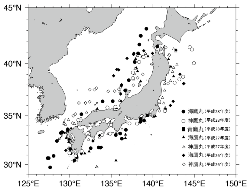
沖合海域のマイクロプラスチック調査の 地点(平成26～28年度の比較)
