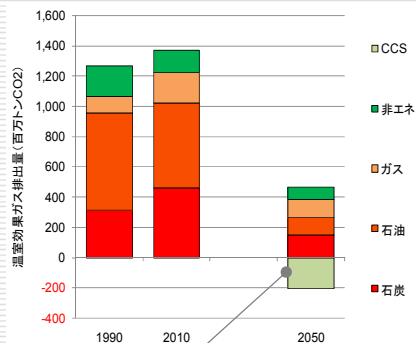
温室効果ガス排出量
