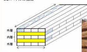
CLTパネルの構成
