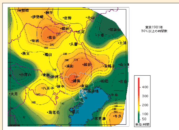
東京地域の高温域の分布: 1981年
