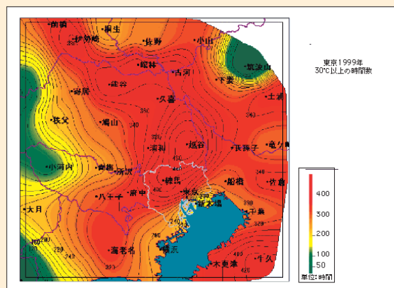
東京地域の高温域の分布: 1999年
