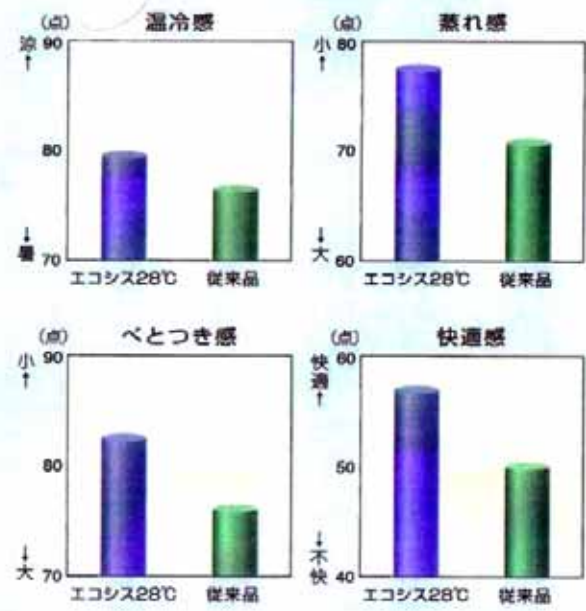
エコシス28℃と従来品の官能評価
