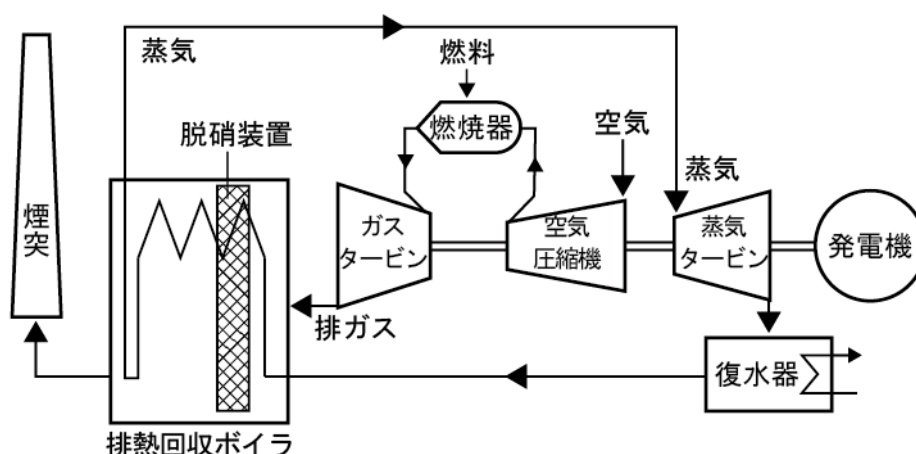
図 1.5-3 GTCC 発電の構造図
