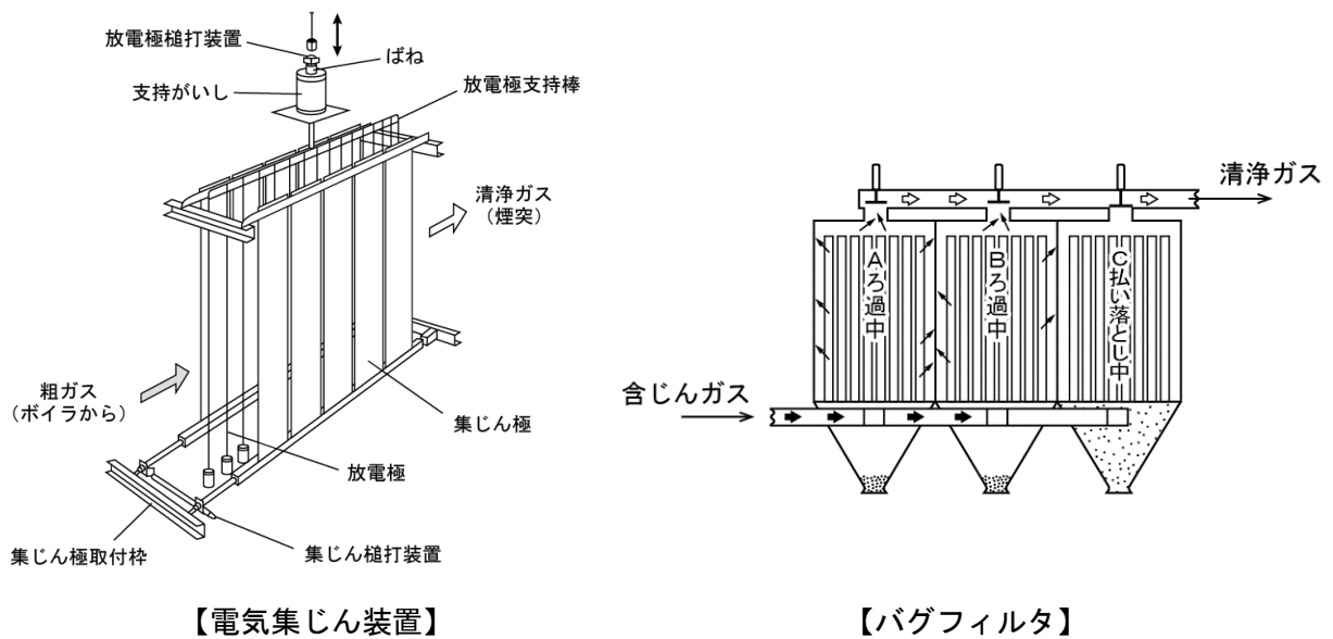
図 2.6-4 集じん装置の概念図
