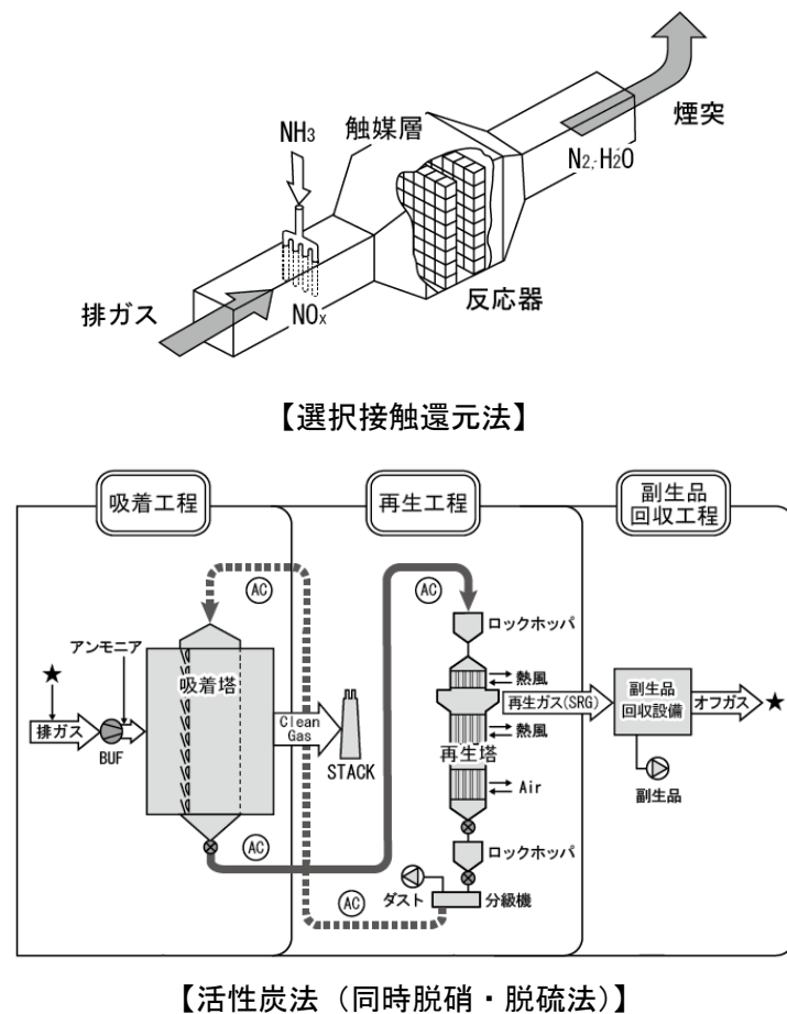
図 2.6-3 排煙脱硝装置の方式別概念図
