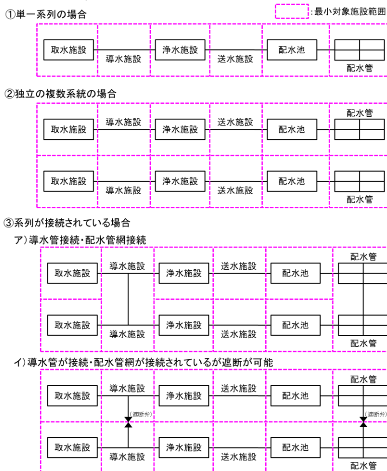
図 2-2 対象となる水道施設の最小範囲の考え方
