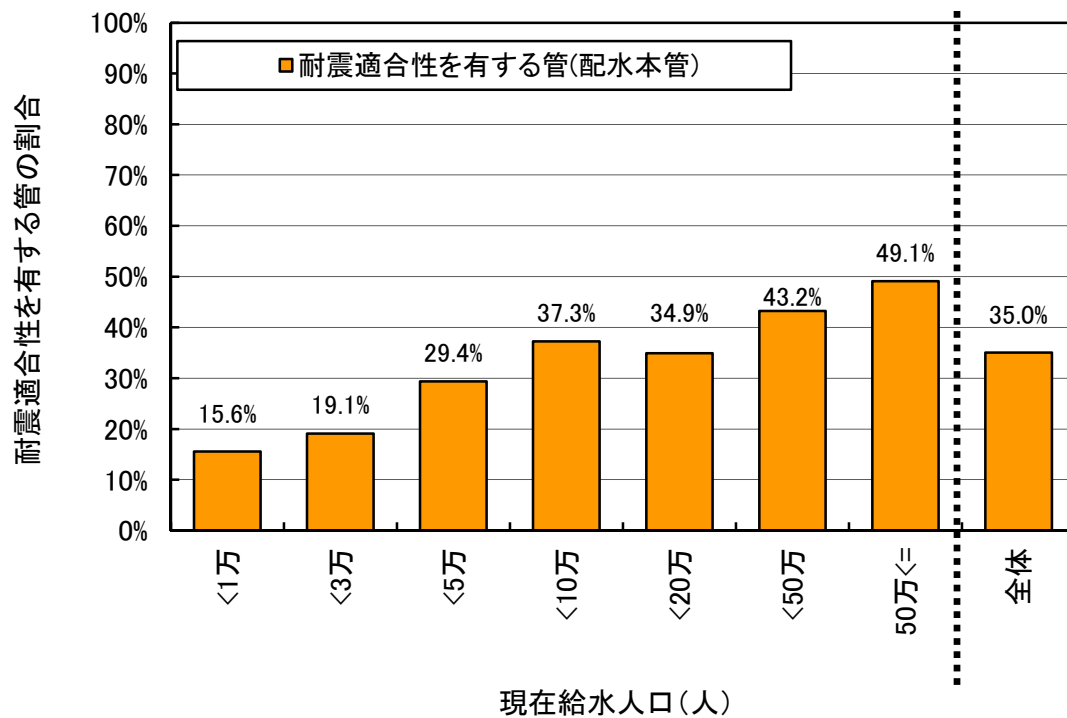
図-3 人口規模別耐震適合性を有する管の割合(配水本管)
