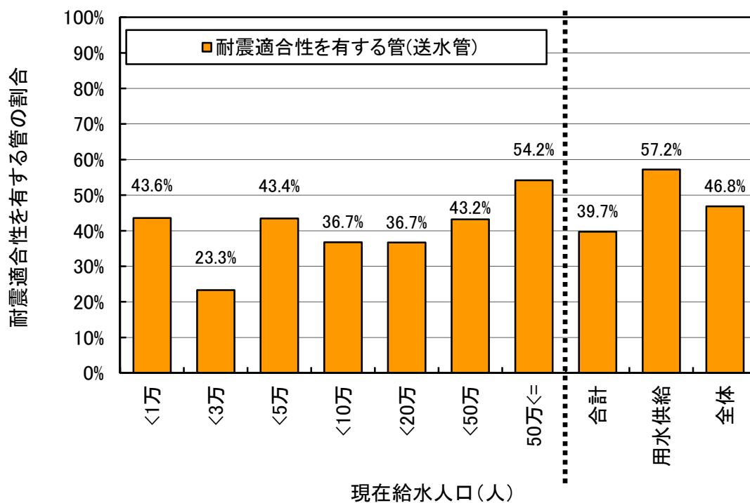
図-2 人口規模別耐震適合性を有する管の割合(送水管)
