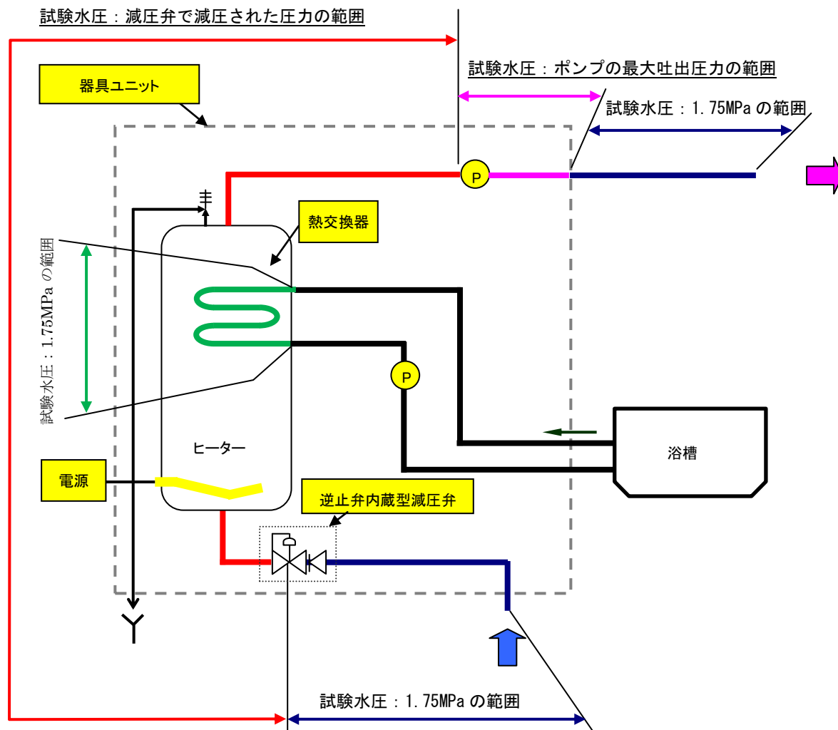
図1-1 改正後の基準省令における耐圧性能試験水压の例
