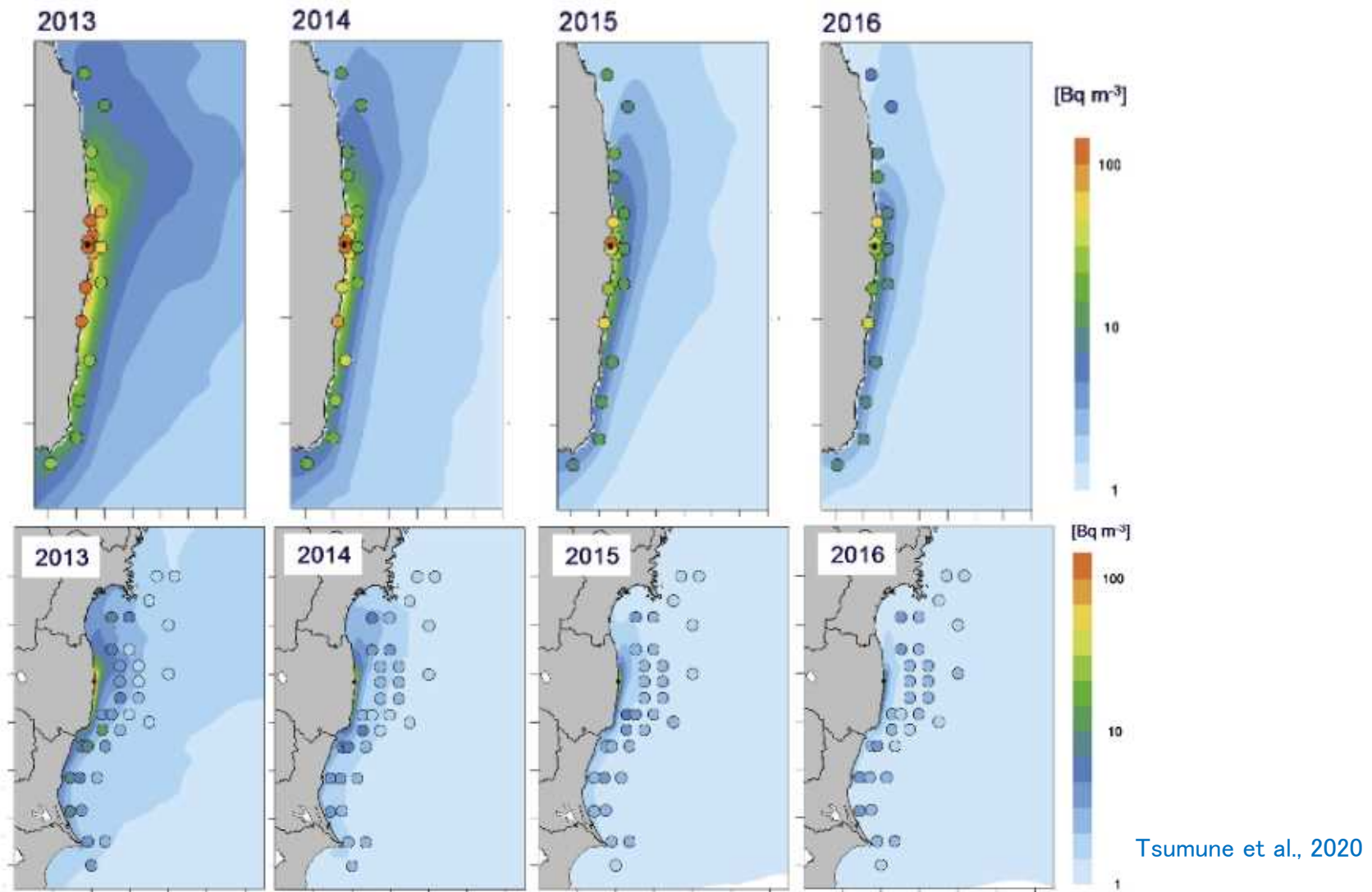
図. 福島沿岸（上）、東北南部～関東北部海域（下）における年平均実測データとシミュレーション結果（2013～2016年） （コンターがシミュレーション、○プロットが実測）
