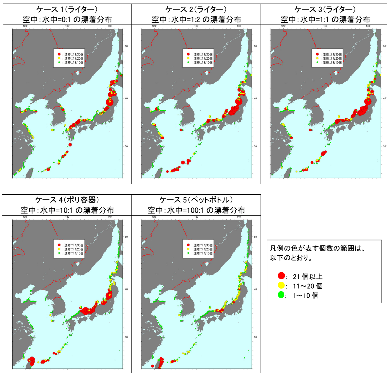
図- 2.41(12) ゴミの漂着分布計算結果(12 月漂着)
