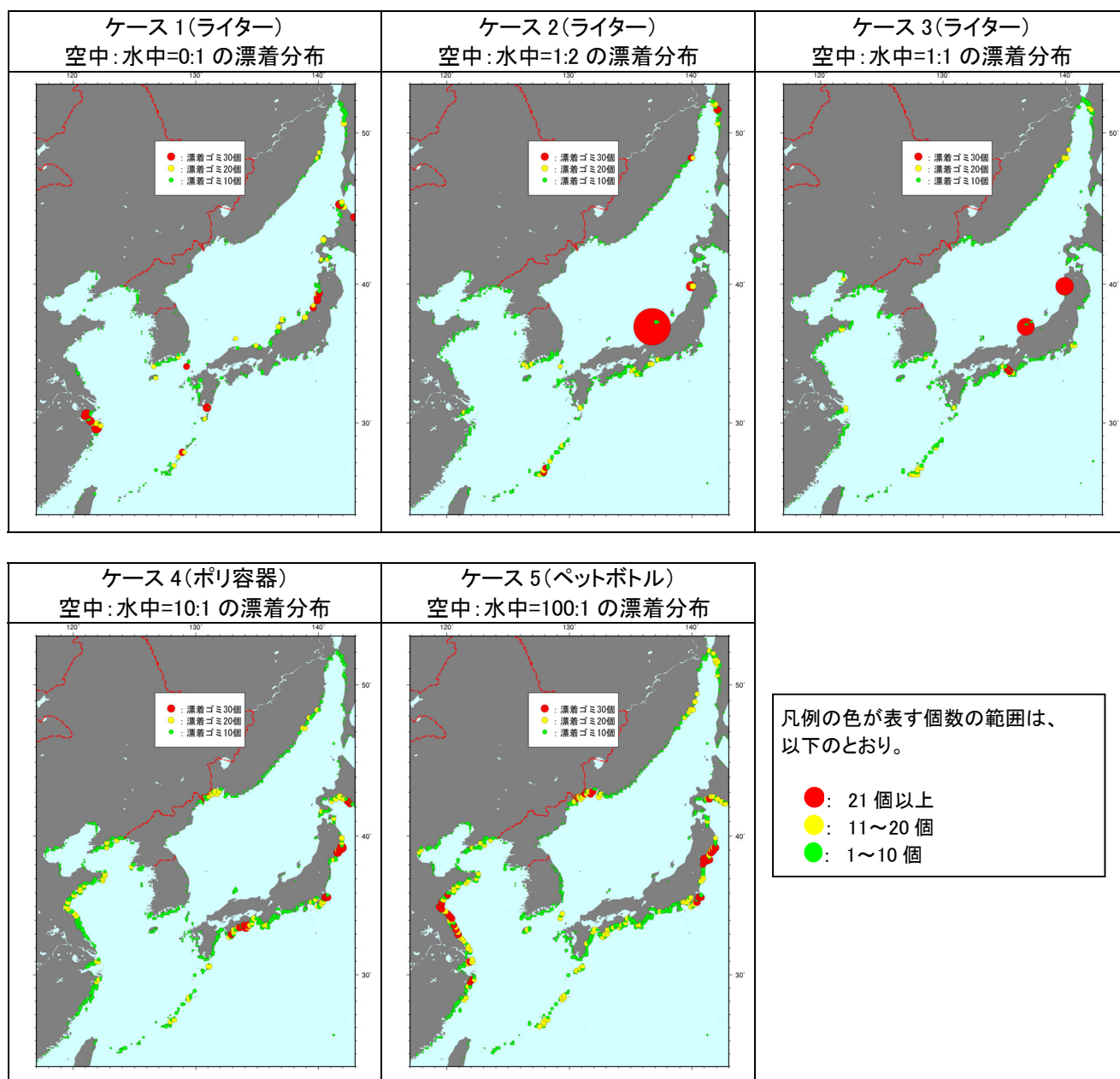
図- 2.41(8) ゴミの漂着分布計算結果(8 月漂着)
