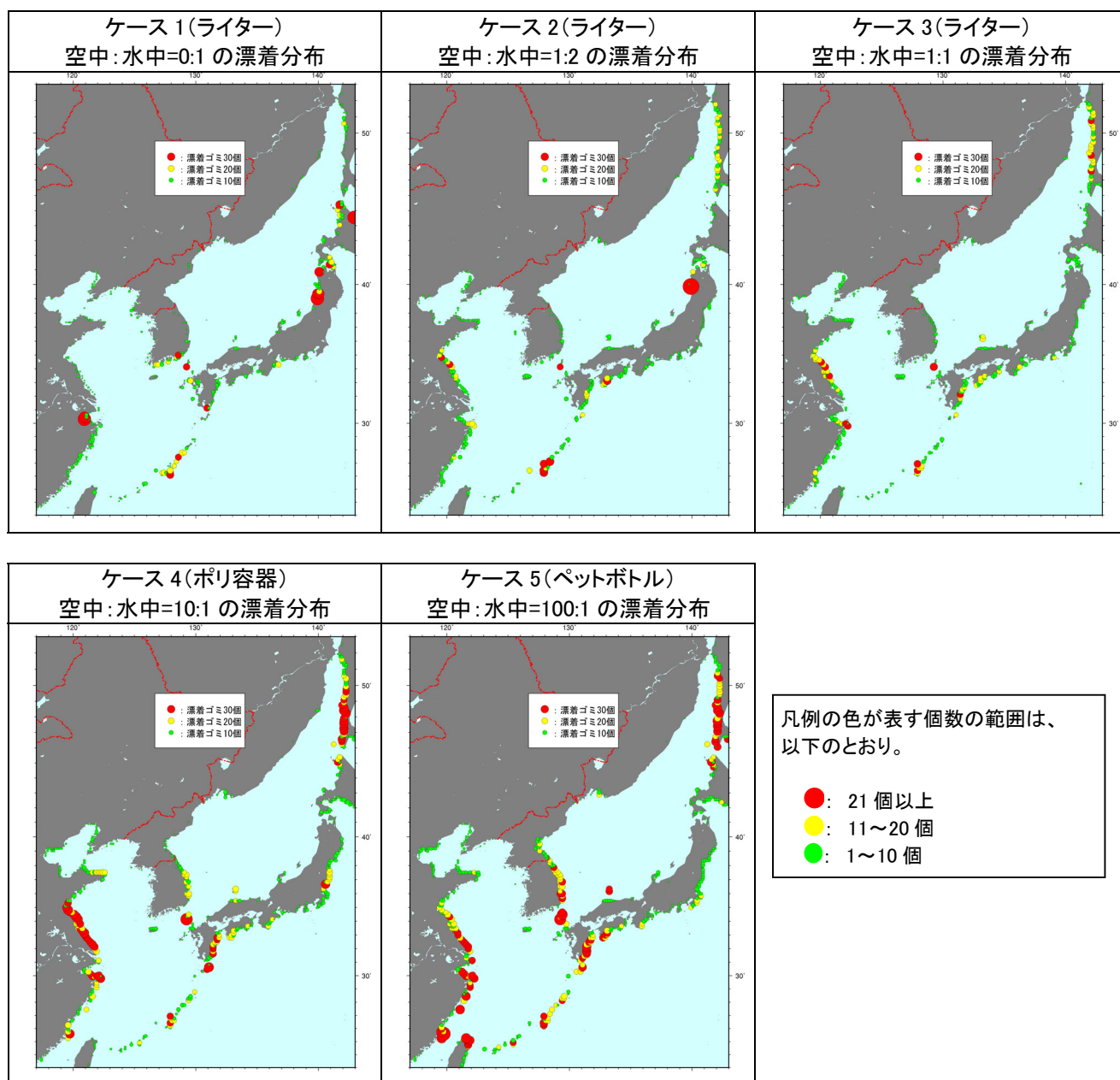
図- 2.41(9) ゴミの漂着分布計算結果(9 月漂着)
