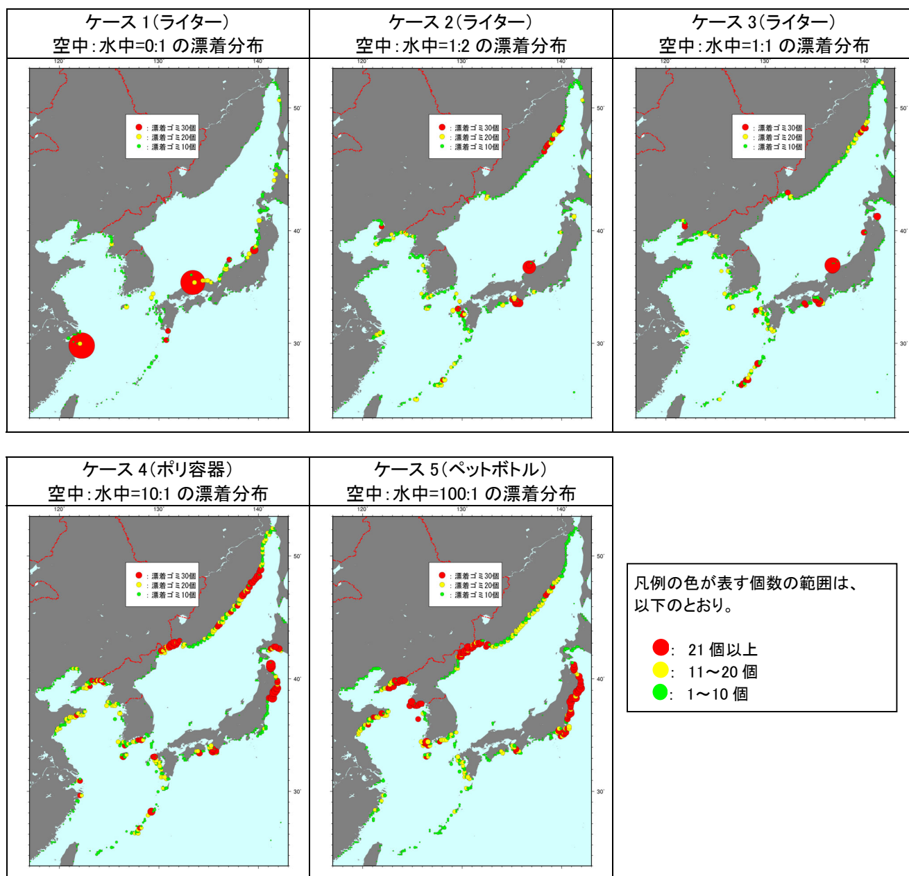
図- 2.41(7) ゴミの漂着分布計算結果(7 月漂着)
