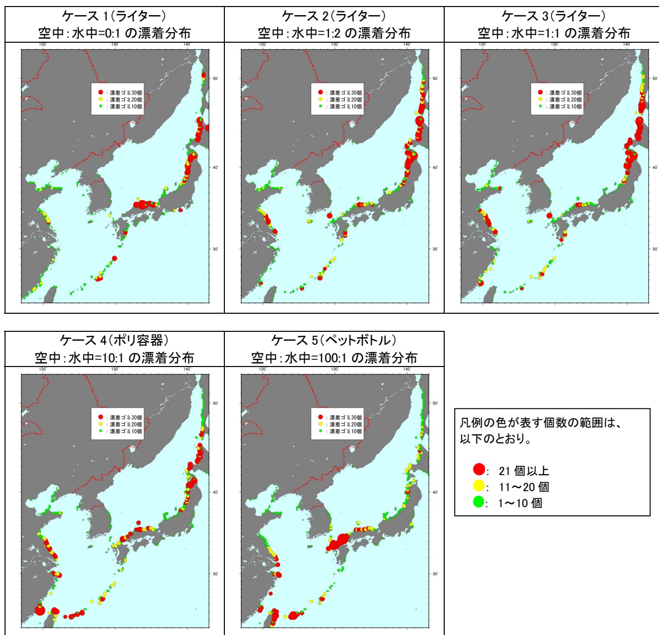
図- 2.41(10) ゴミの漂着分布計算結果(10 月漂着)
