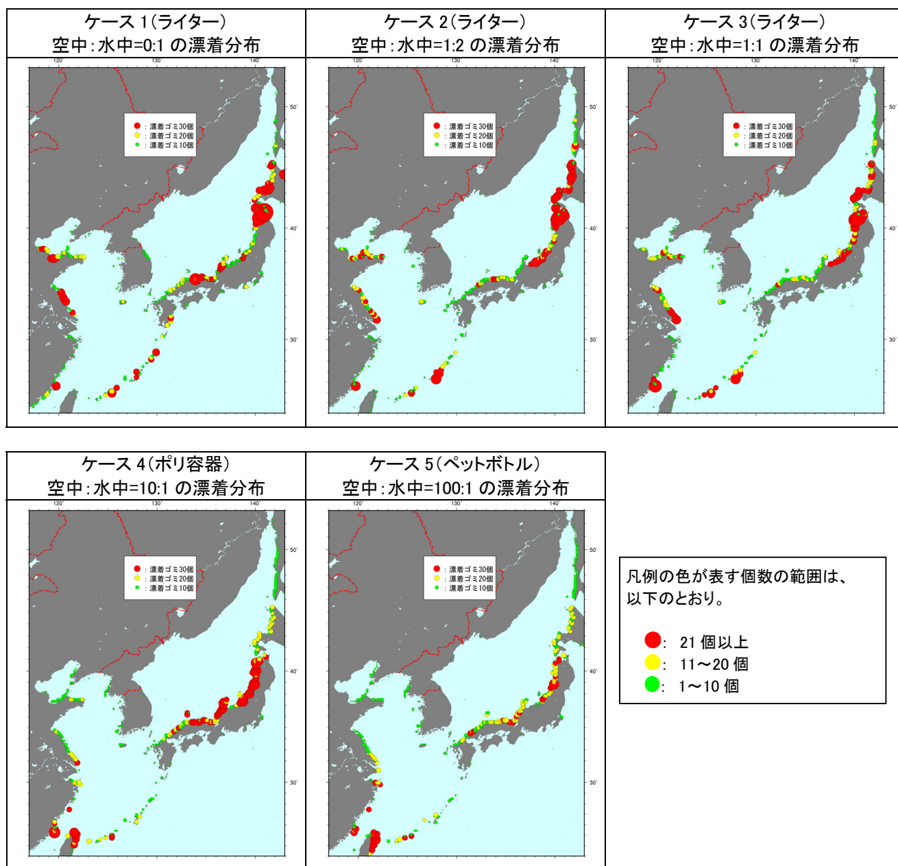
図- 2.41(11) ゴミの漂着分布計算結果(11 月漂着)
