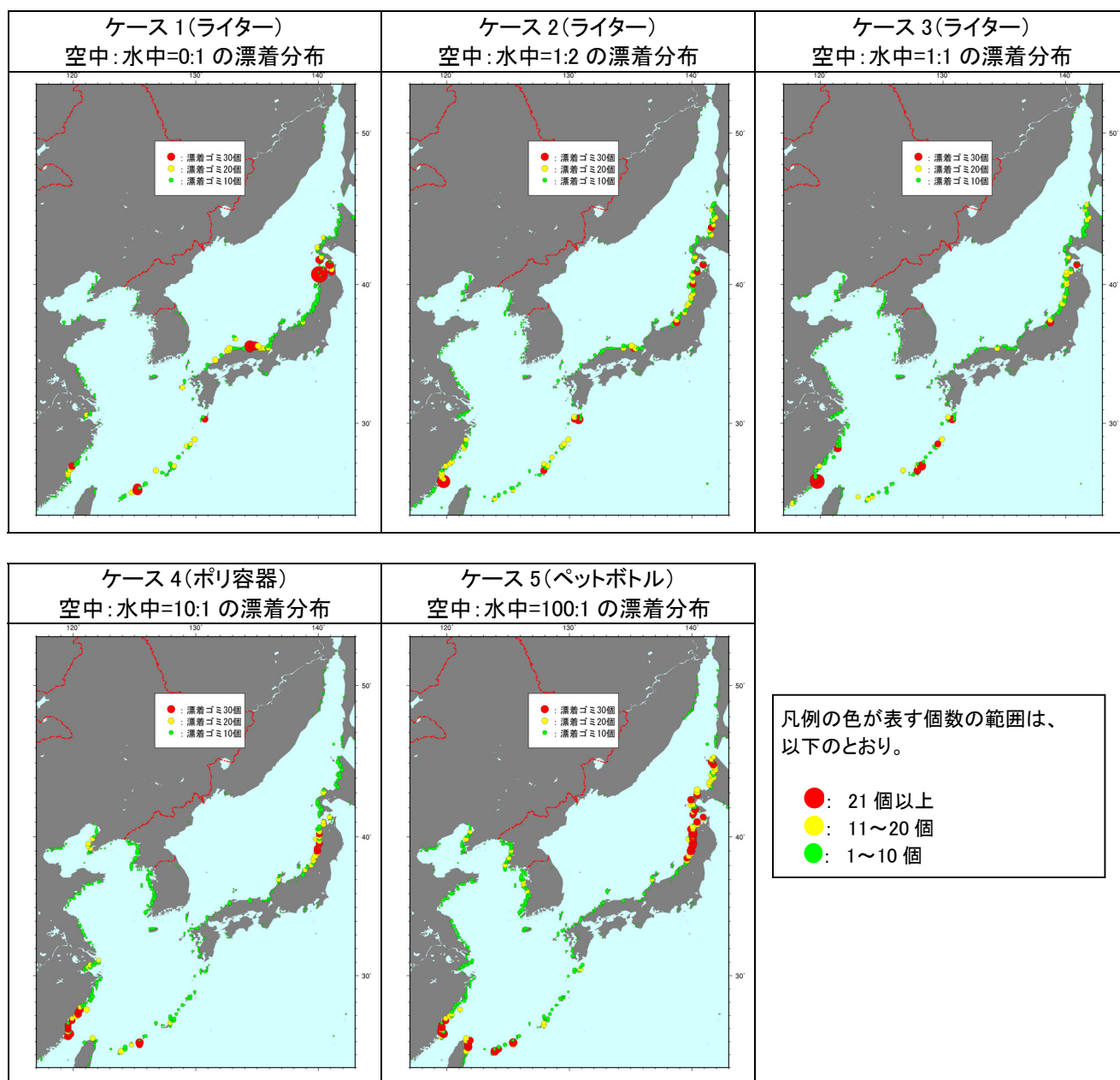
図- 2.41(4) ゴミの漂着分布計算結果(4 月漂着)
