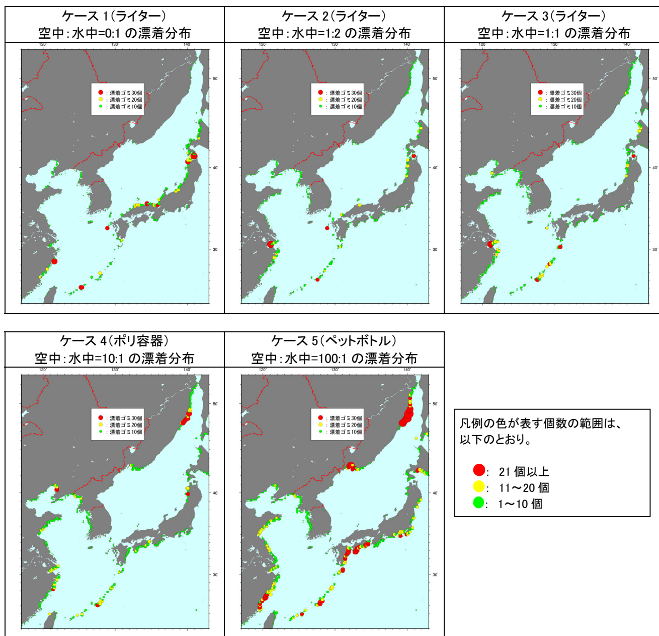
図- 2.41(5) ゴミの漂着分布計算結果(5 月漂着)
