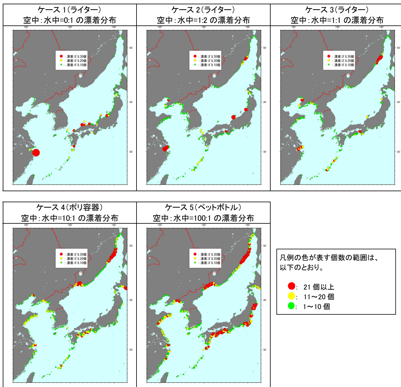
図- 2.41(6) ゴミの漂着分布計算結果(6 月漂着)
