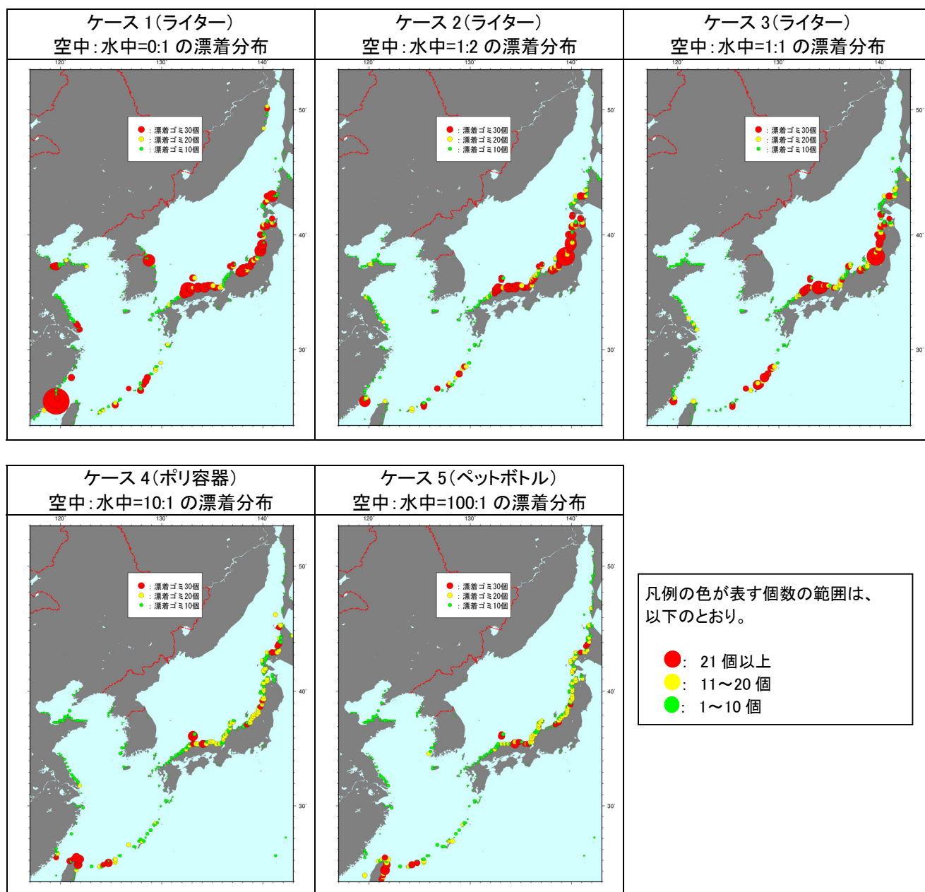
図- 2.41(1) ゴミの漂着分布計算結果(1 月漂着)
