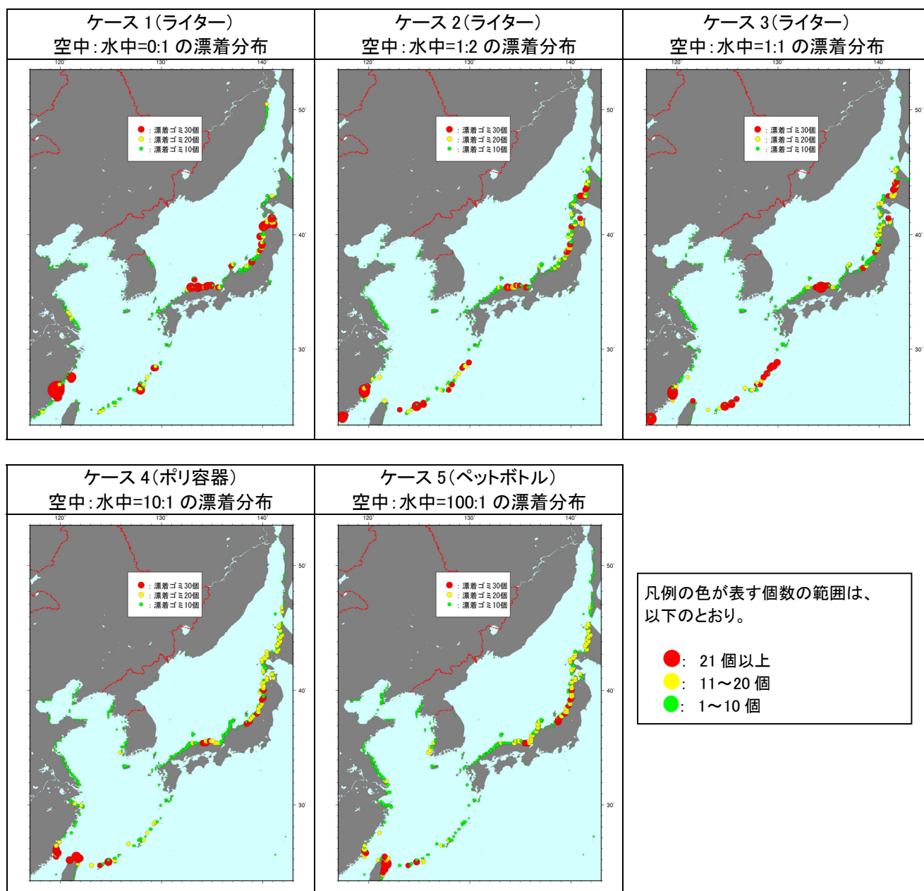
図- 2.41(3) ゴミの漂着分布計算結果(3 月漂着)
