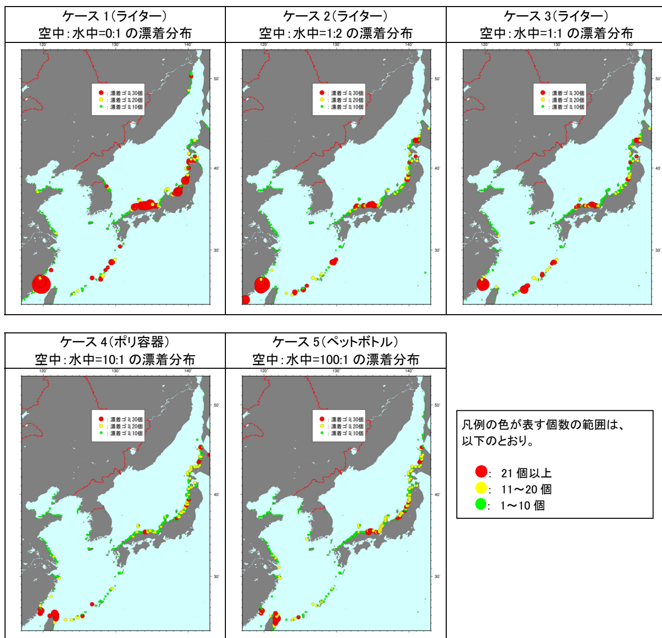
図- 2.41(2) ゴミの漂着分布計算結果(2 月漂着)
