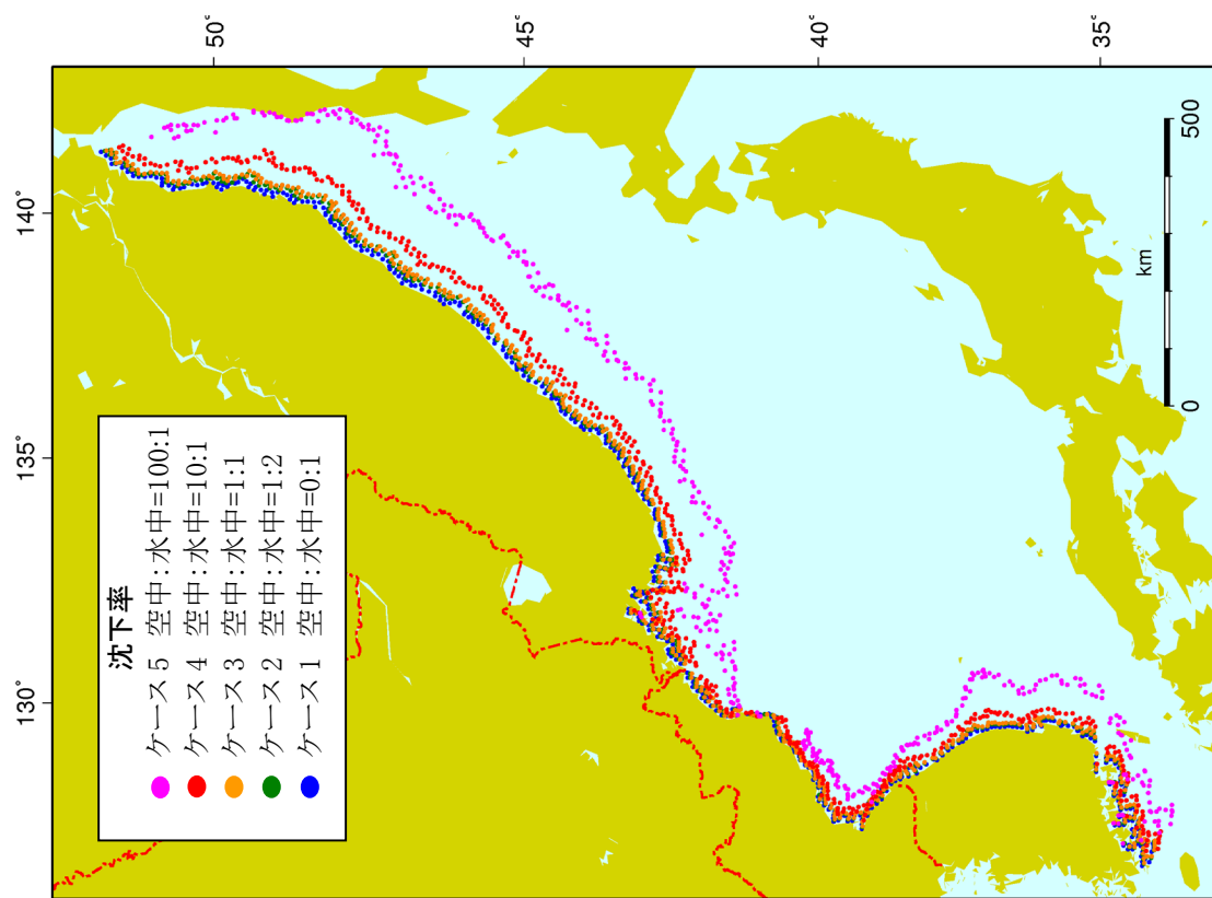
図-2.30(1) 計算開始 1 日後の漂流分布
