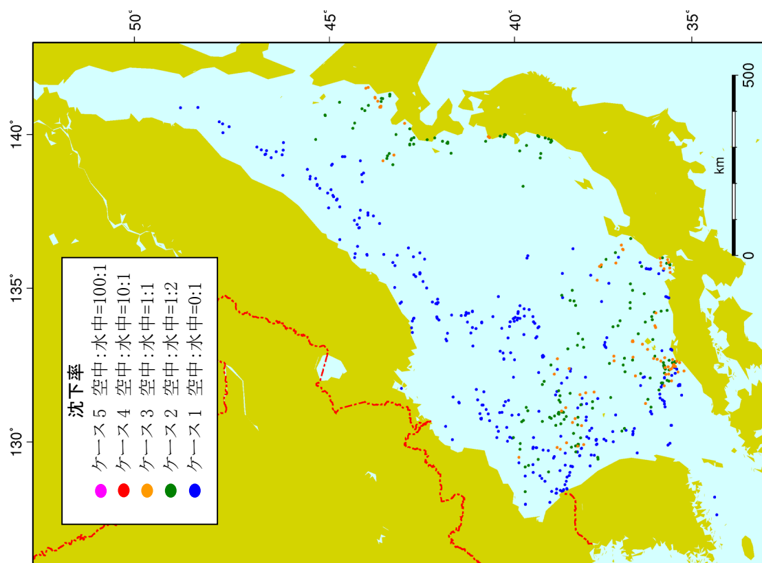
図-2.30(8) 計算開始 60 日後の漂流分布
