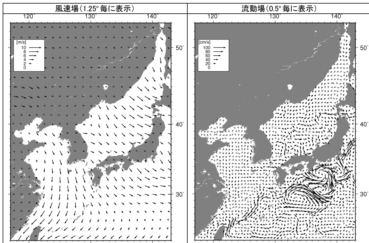
図- 2.37(2) 2 月の風速場と流動場
