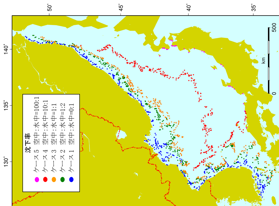
図-2.30(4) 計算開始 10 日後の漂流分布
