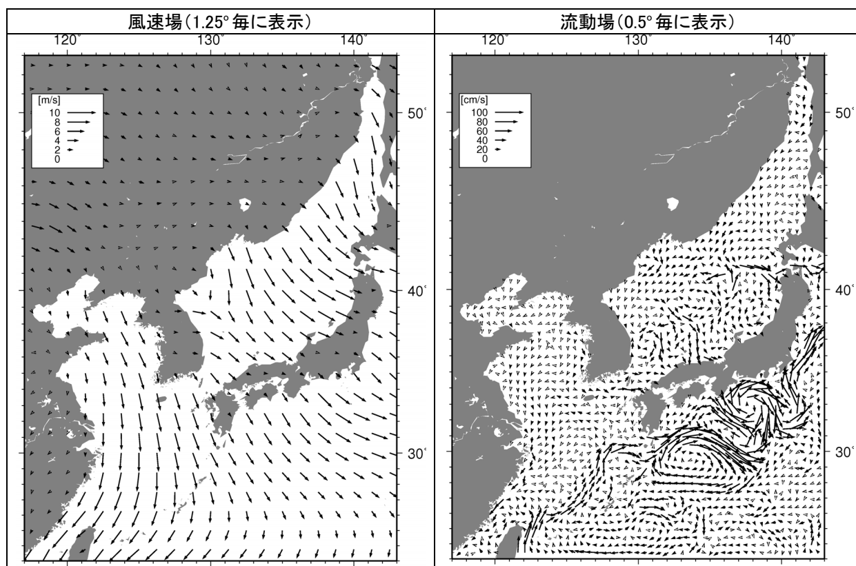
図- 2.37(1) 1 月の風速場と流動場
