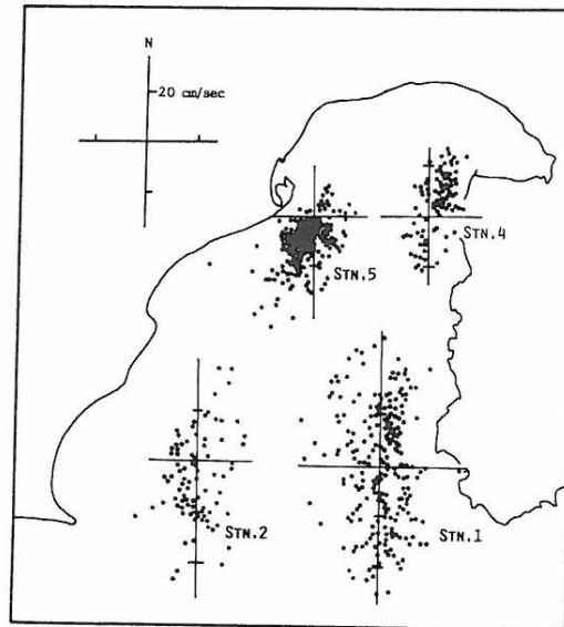
図V-7 駿河湾内4地点における25時間ベクトル平均値散布図
