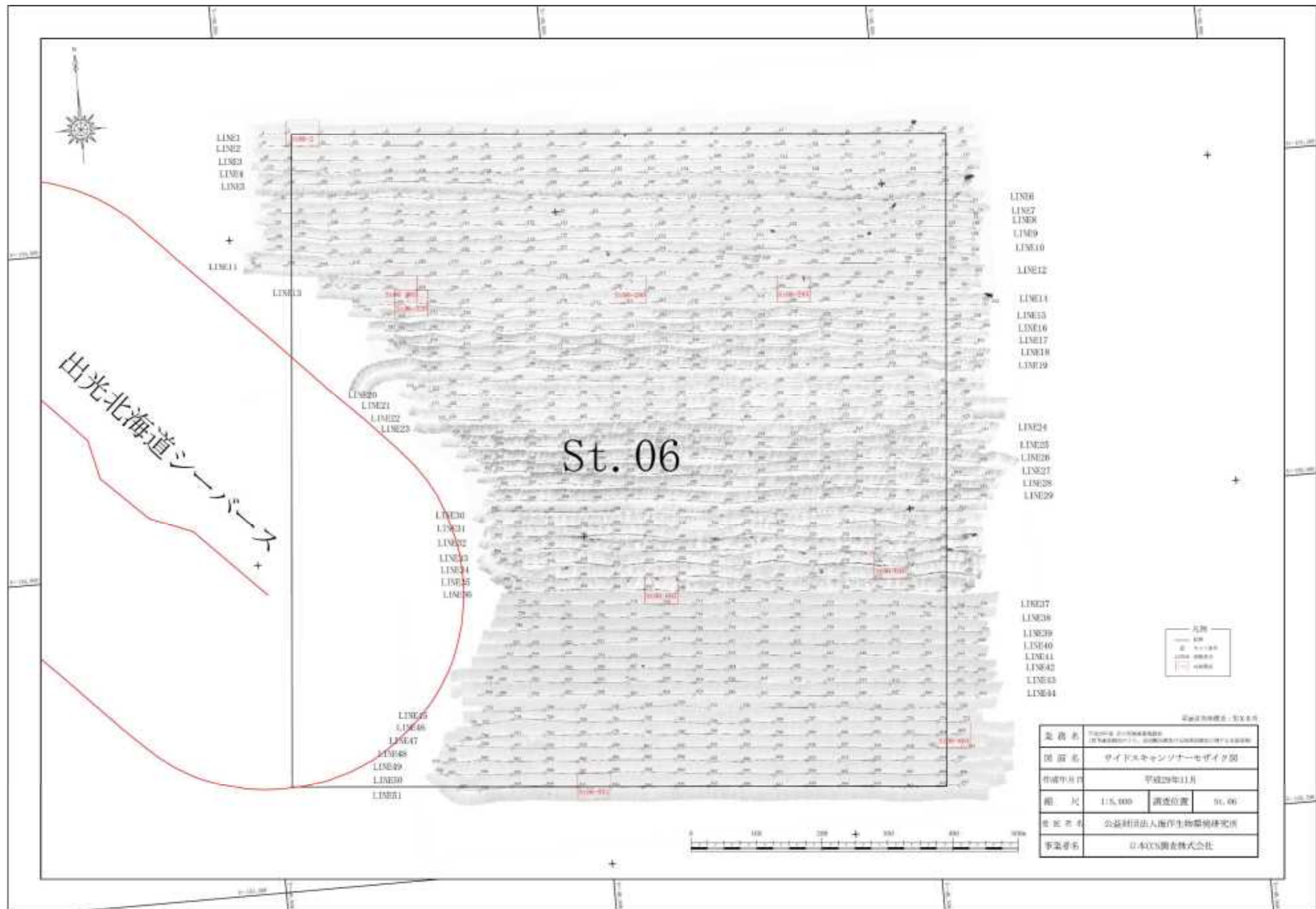
第 4.3.6 図 St. 06 の気泡確認調査におけるサイドスキャンソナーモザイク図（シーバースから約 300m の区域と重なる測線は、調査を実施していない）
