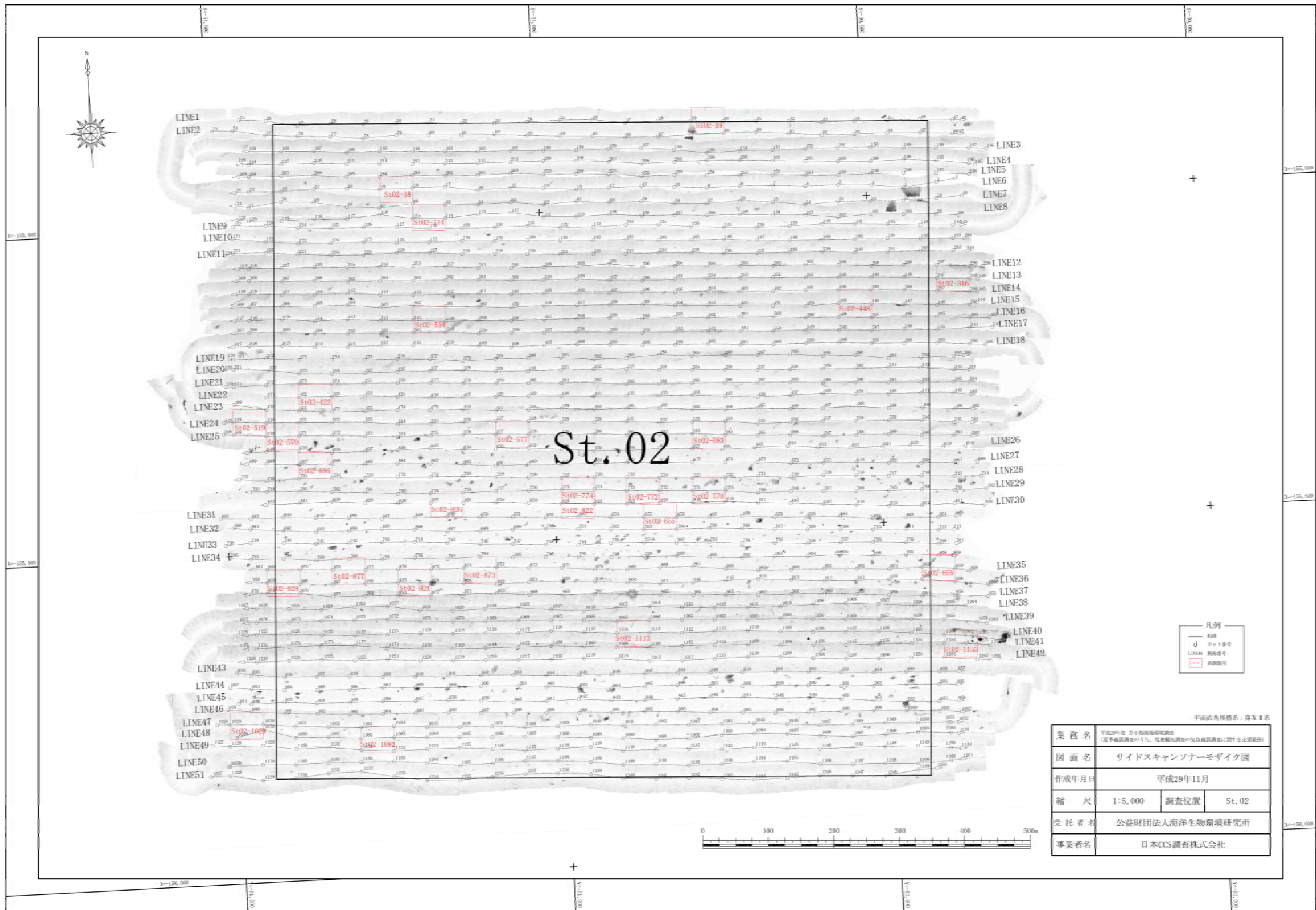
第 4.3.4 図 St. 02 の気泡確認調査におけるサイドスキャンソナーモザイク図
