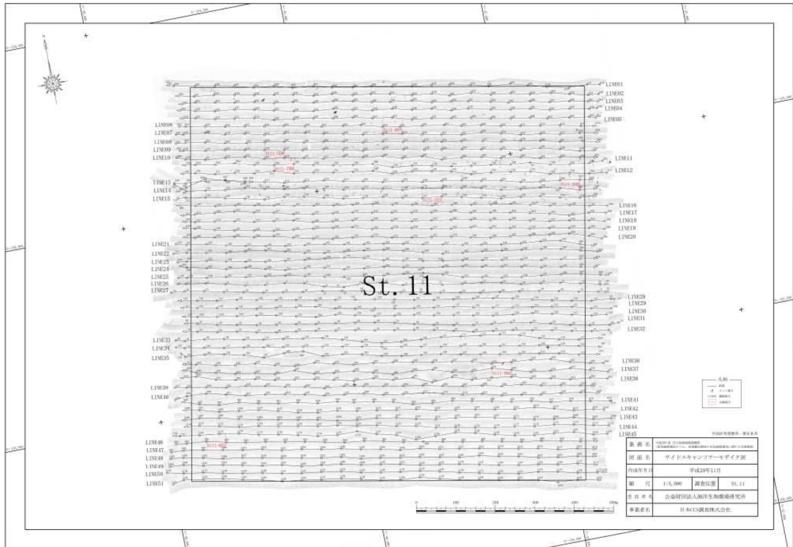
第 4.3.7 図 St. 11 の気泡確認調査におけるサイドスキャンソナーモザイク図
