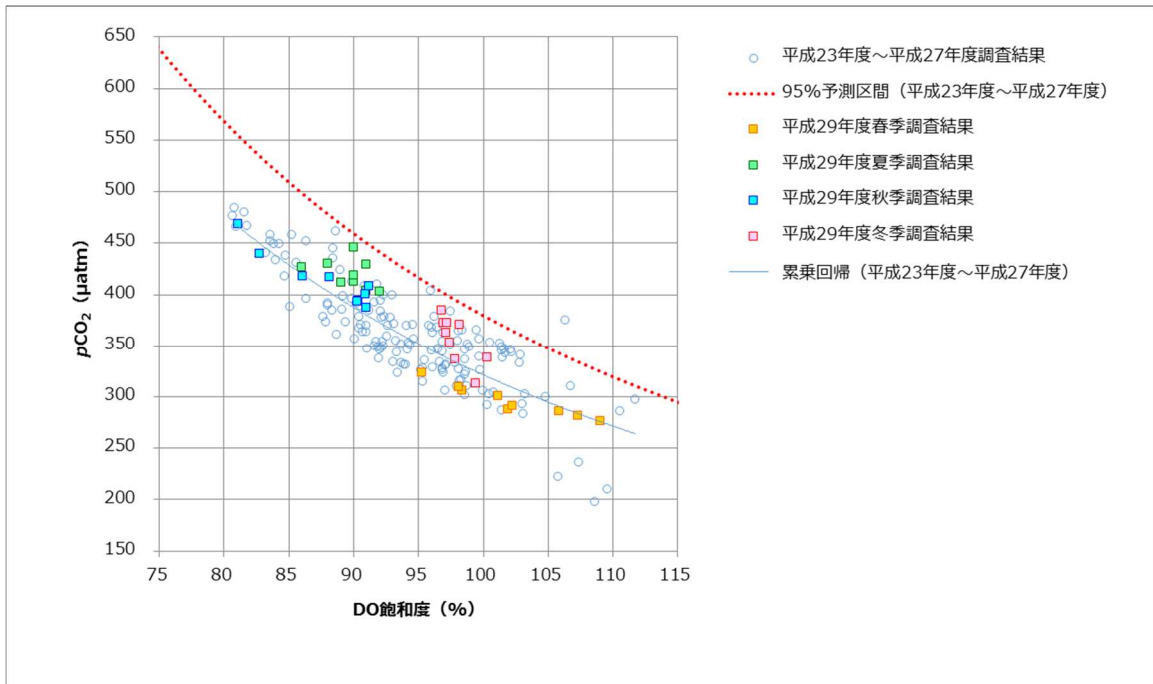
参考図 pCO_2 と DO 飽和度との関係 (平成 29 年度調査結果)
