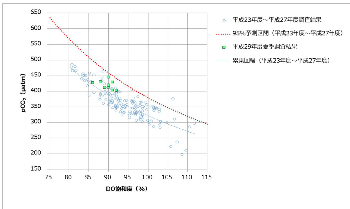
図5 pCO 2 と DO 飽和度との関係
