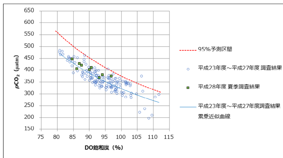
図 5 p\text{CO}_2 と DO 飽和度との関係
