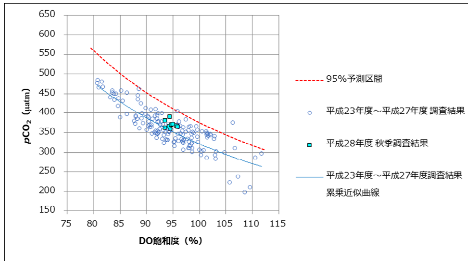
図5 pCO 2 とDO飽和度との関係
