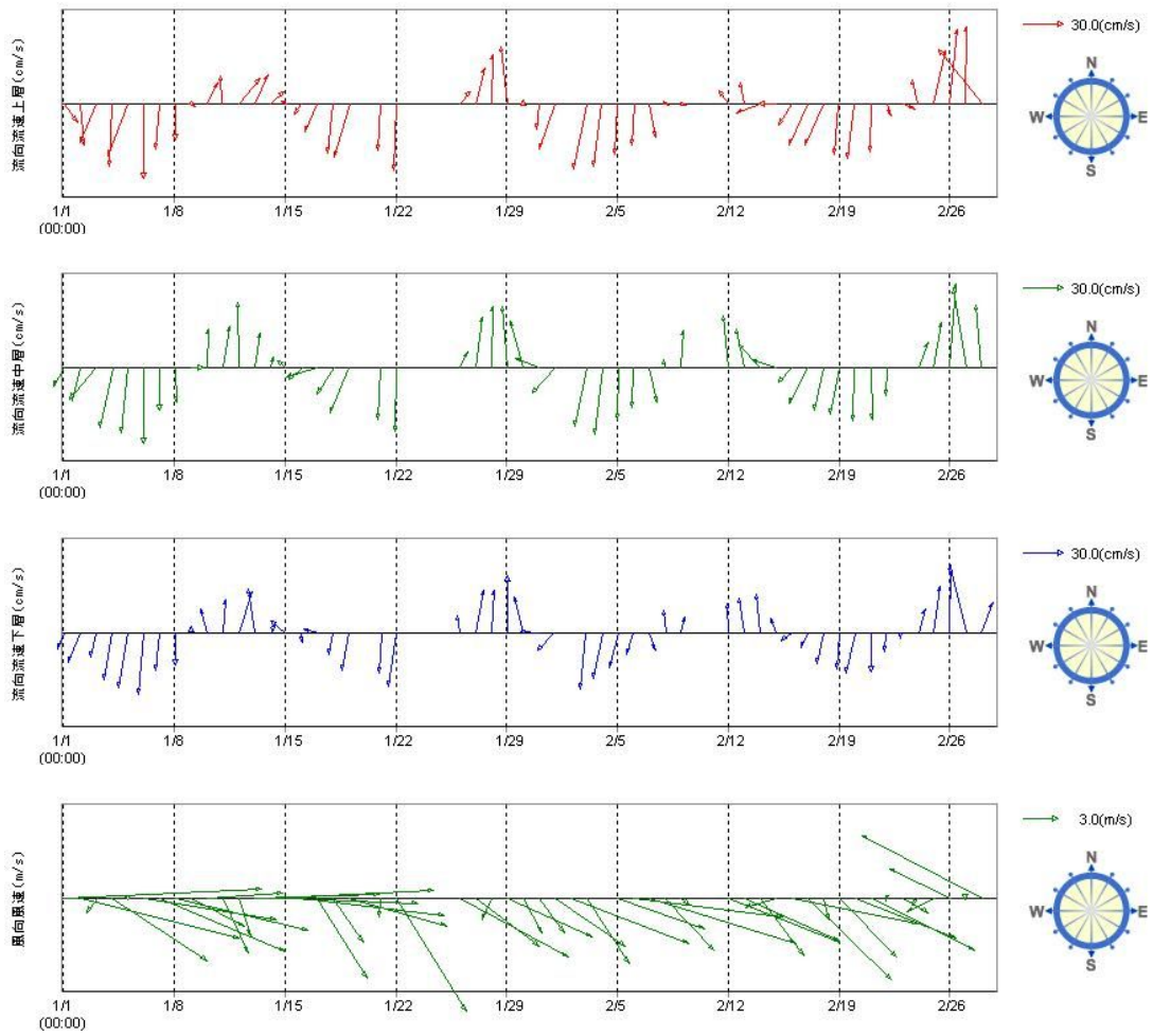
図 2.5.7(2) 三河湾湾口(中山水道)における観測データ(2010年1~2月)
