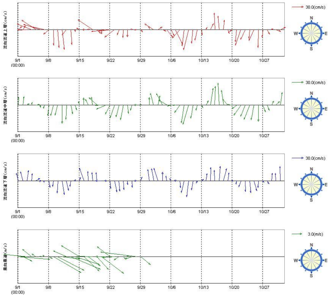
図 2.5.5(2) 三河湾湾口(中山水道)における観測データ(2009年9~10月)
