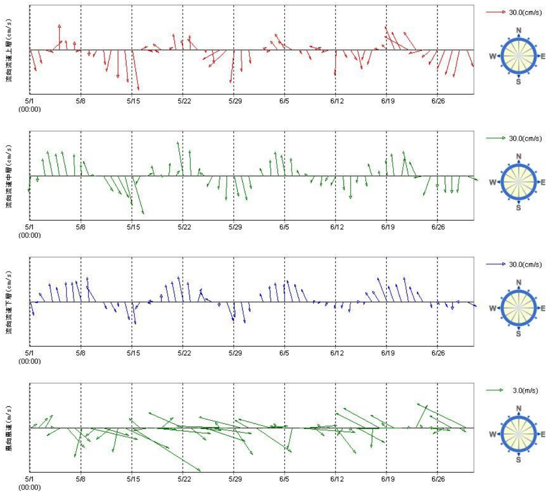
図 2.5.3(2) 三河湾湾口(中山水道)における観測データ(2009年5~6月)
