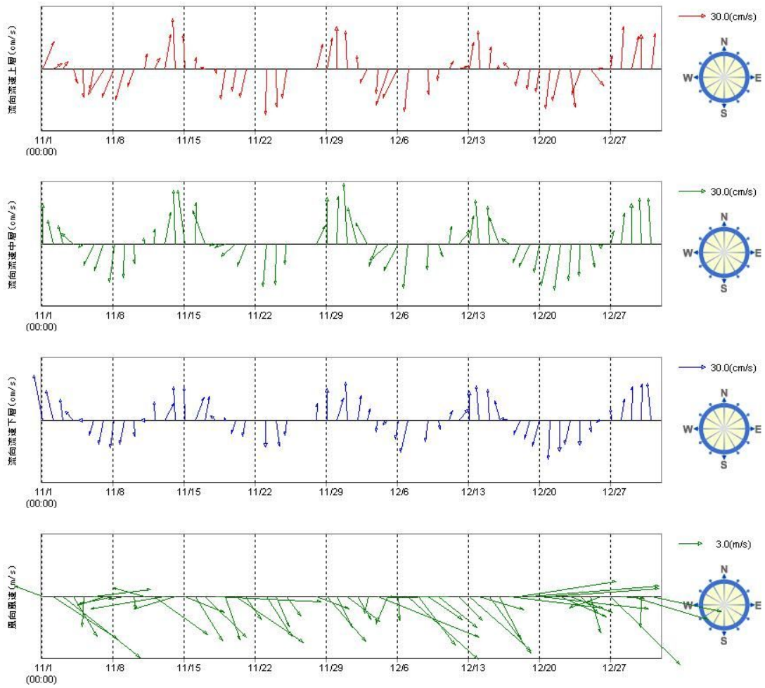
図 2.5.6(2) 三河湾湾口(中山水道)における観測データ(2009年11~12月)
