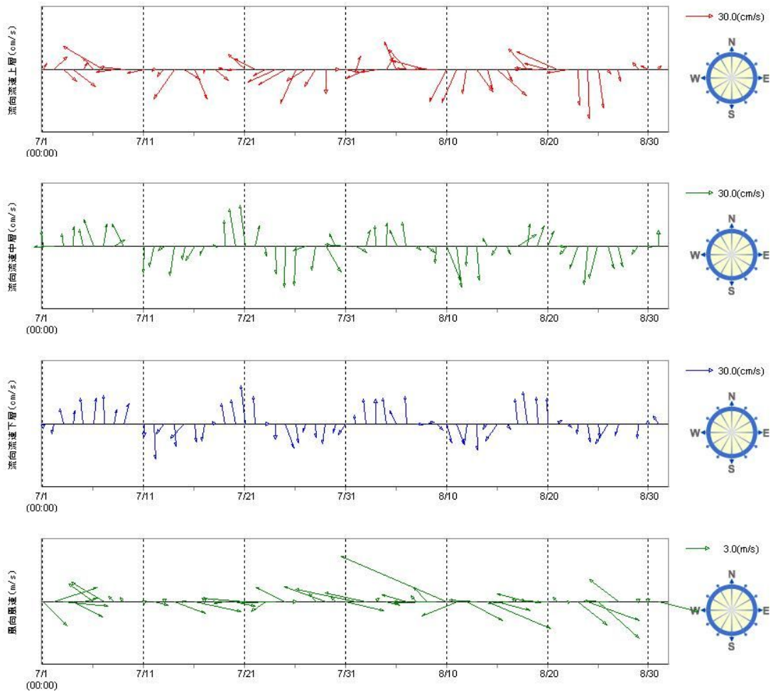
図 2.5.4(2) 三河湾湾口(中山水道)における観測データ(2009年7~8月)
