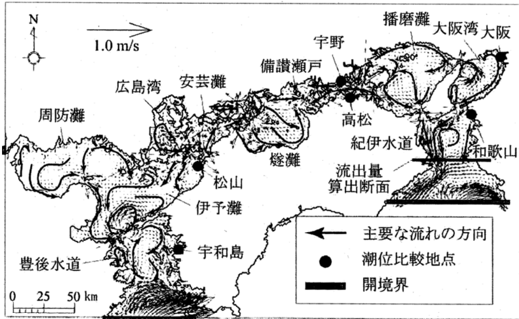
図 3.9 (2) 恒流図、中山(2011)による
