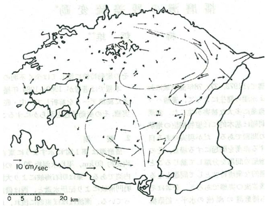
図 3.9 (4) 恒流図、柳(1986)による
