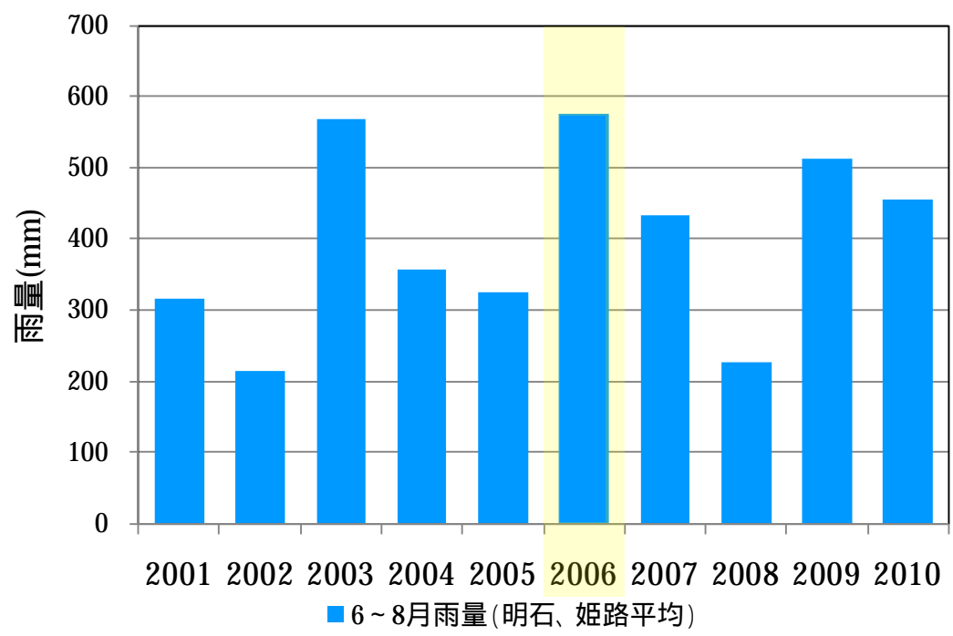
図 3.10 明石、姫路における6~8月の年別雨量
