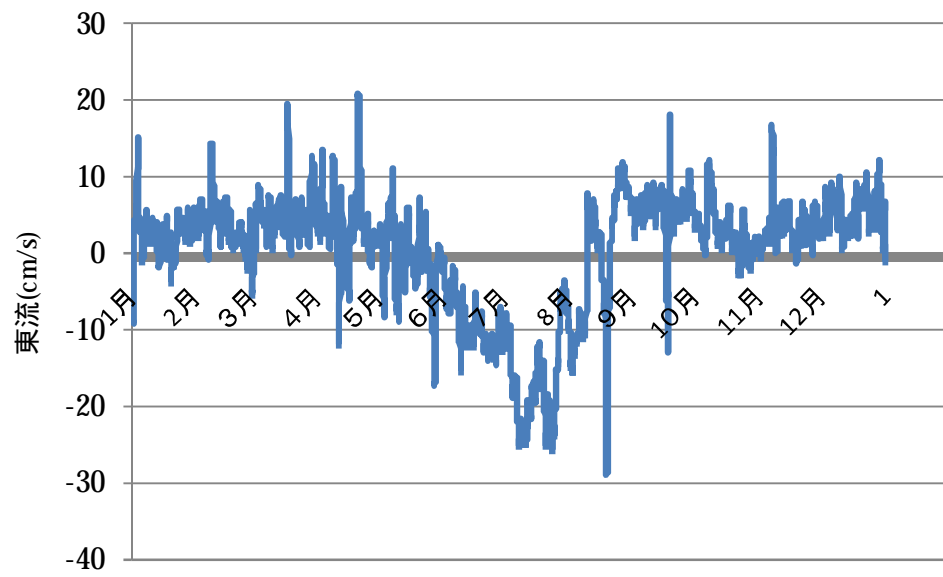
図 3.11 明石沖における 25 時間移動平均東西流
