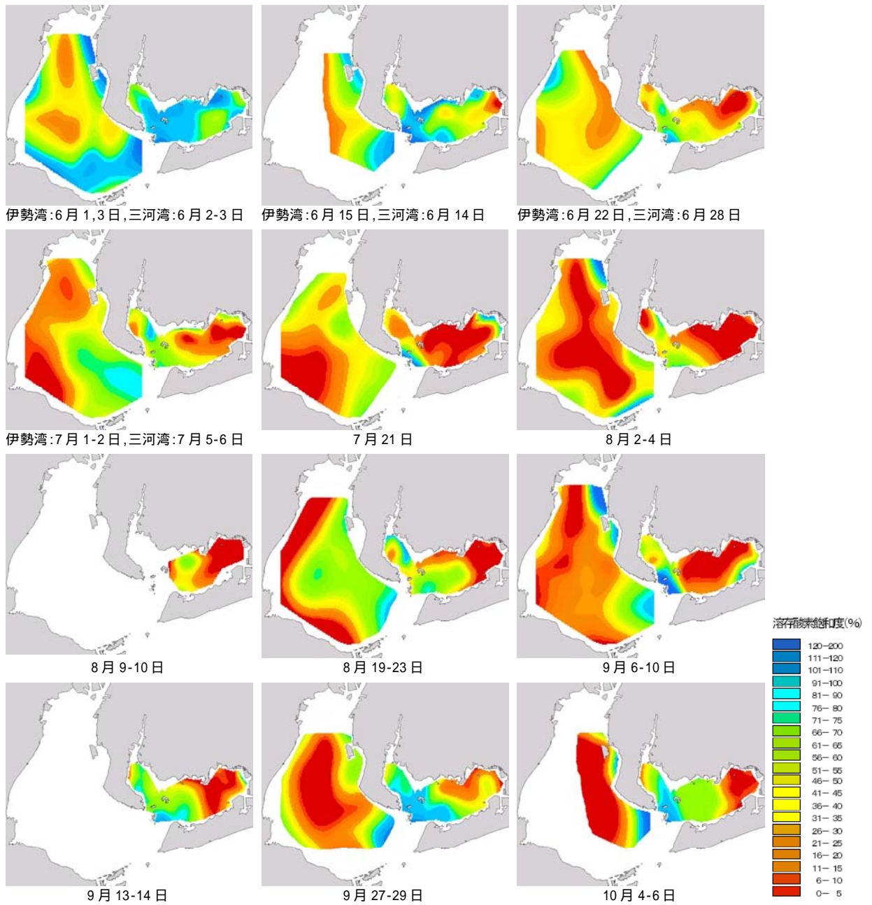
図 2.13 三河湾の底層溶存酸素飽和度分布 (2010年) (愛知県水産試験場ホームページより)
