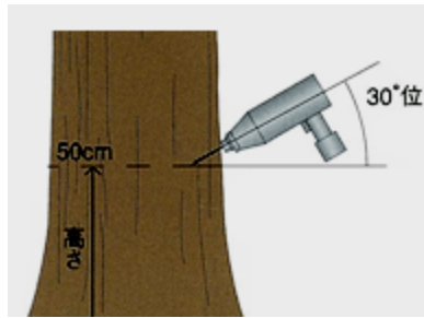
図6. 樹幹注入の例 ( http://www.greenguard.jp/product/ )
