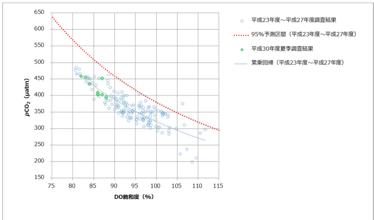
図 5 p\text{CO}_2 と DO 飽和度との関係
