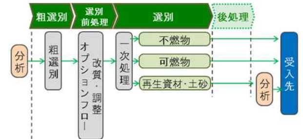
選別処理主体の処理フローのケースの例
