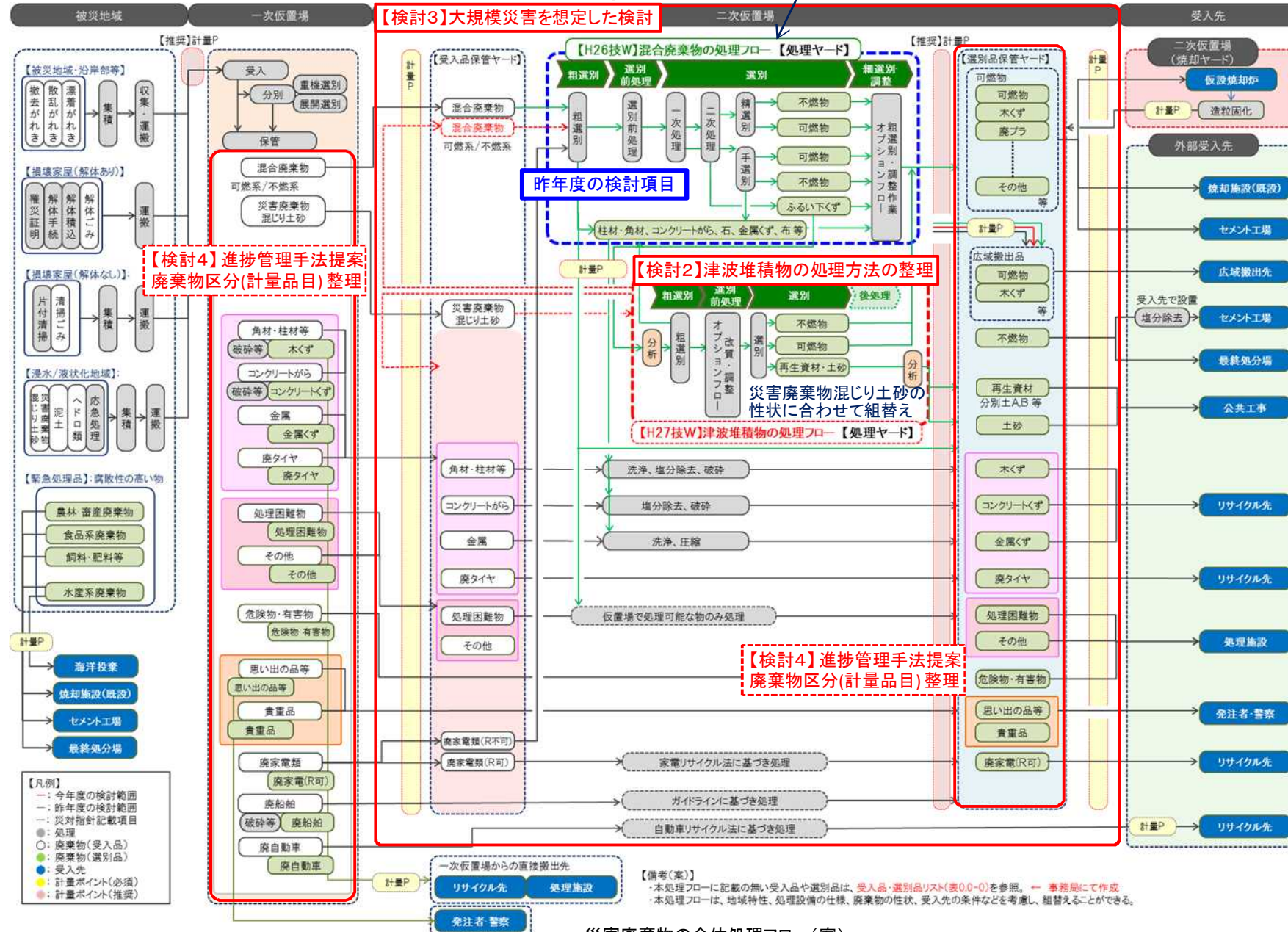
災害廃棄物の全体処理フロー(案)
