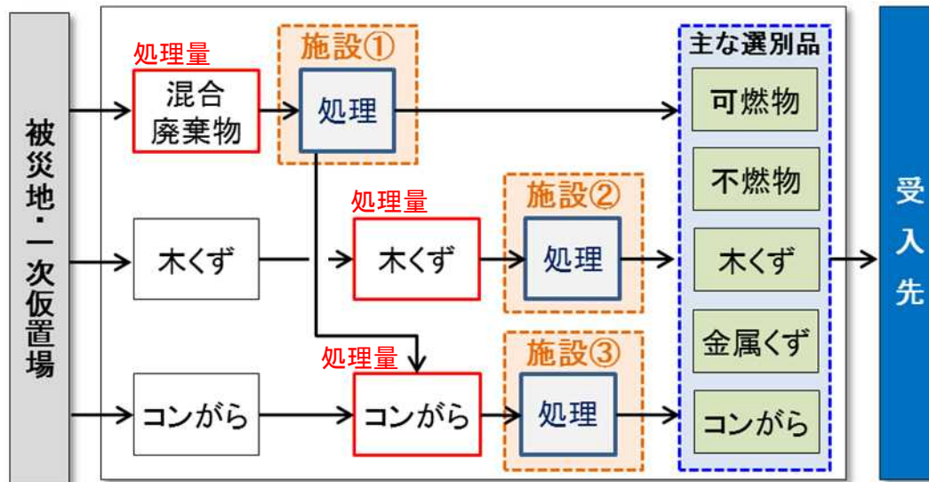
処理フローの例(混合廃棄物・木くず・コンガラ)
