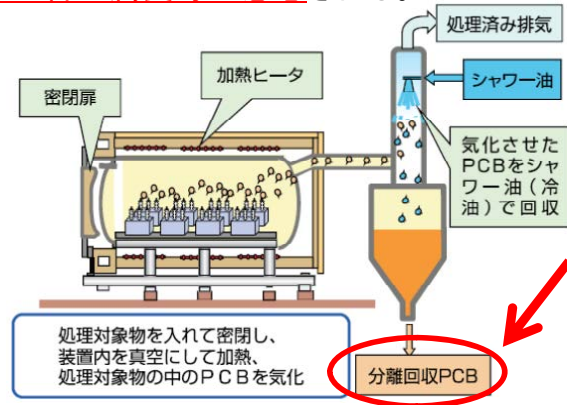
真空加熱分離の概要
