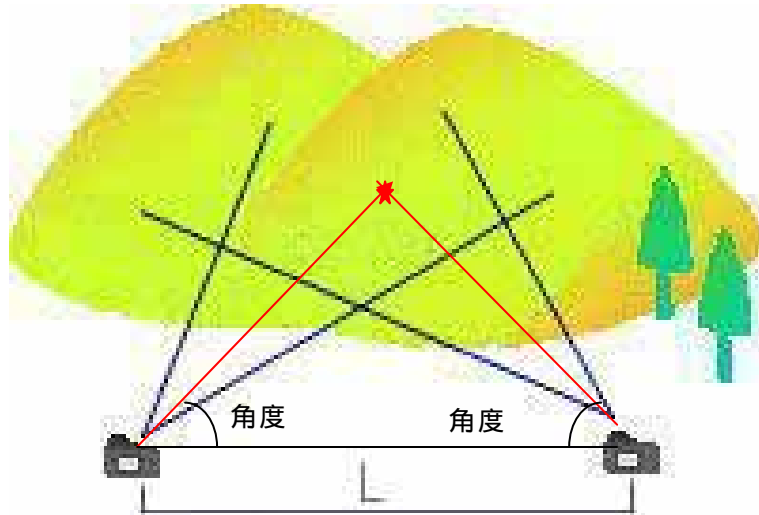
図 3 写真測量の概念
