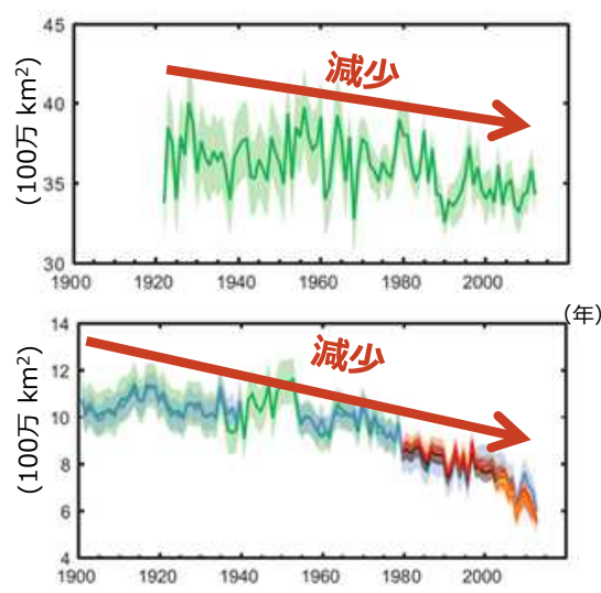
図.北半球積雪面積の変化（春季）（上）（年） 北極域海氷面積の変化（夏季）（下）
