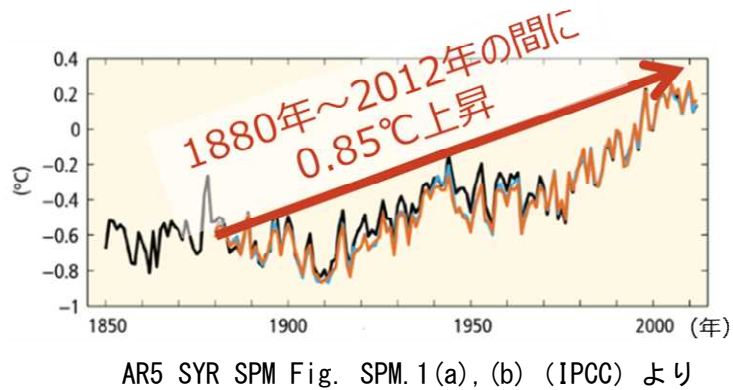
図1 陸域と海上を合わせた世界平均地上気温偏差の変化
