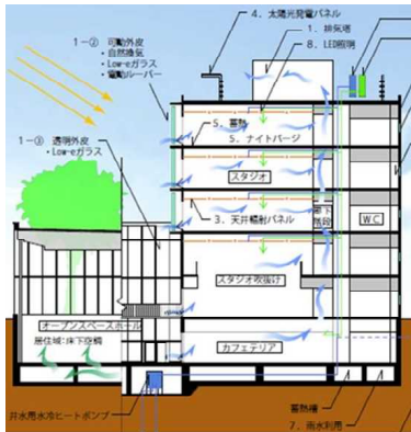
【省エネ化された住宅・建築物】
