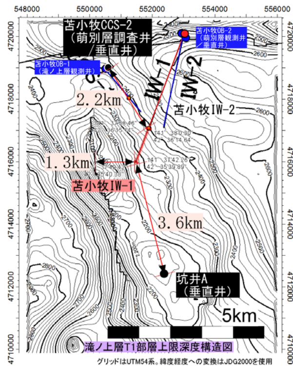
第 6. 1-2 図 潜ノ上層圧入井周辺の圧入した CO 2 の分布予測範囲と、周辺の断層および廃坑井との位置関係
