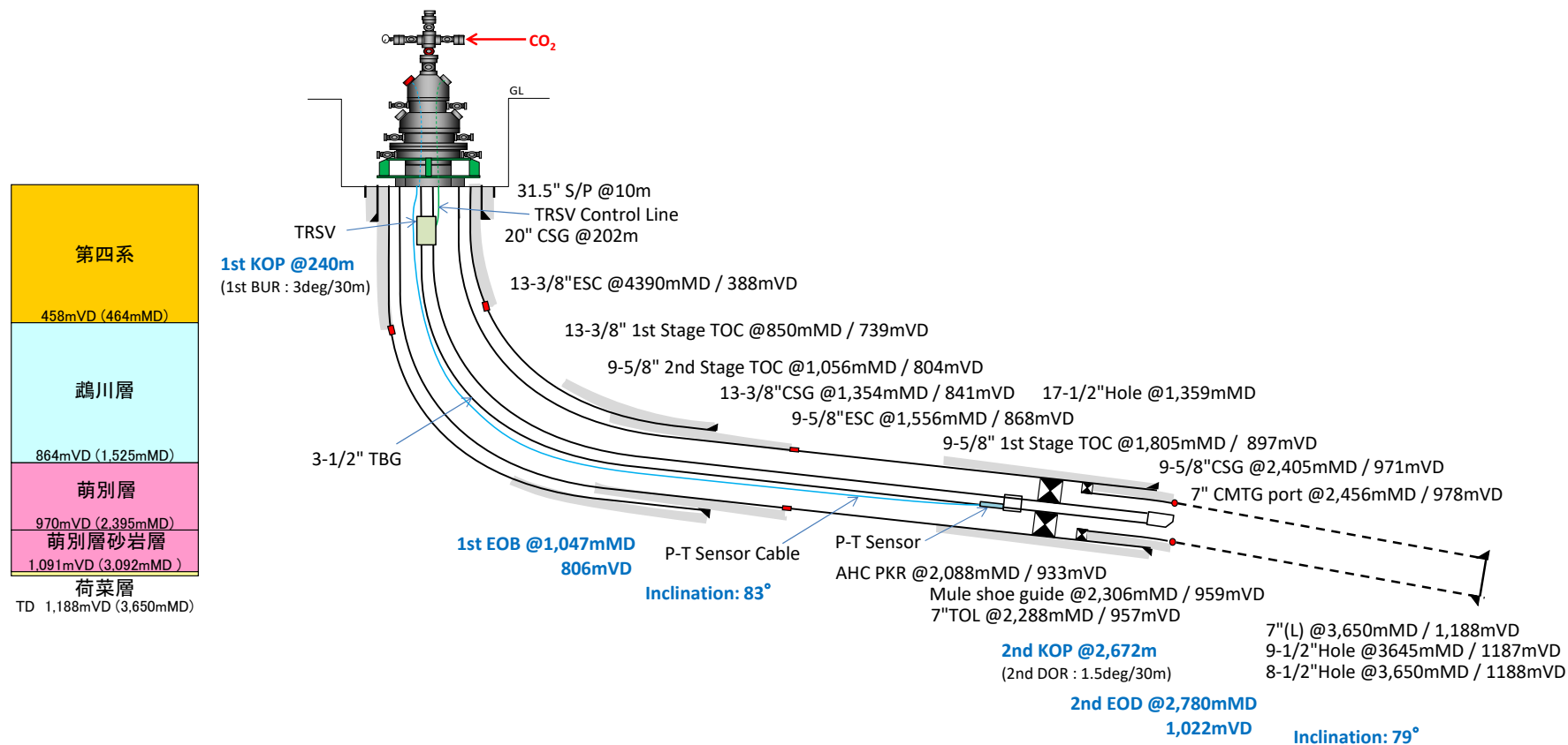
第 5.4-2 図 萌別層圧入井の坑内
