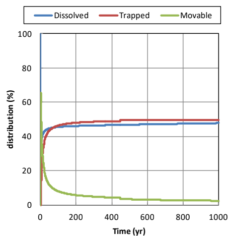
第 4.5-45 図 低浸透率ケースにおける CO 2 の貯留フォーム（割合）の変化（平成 23 年度シミュレーション結果）
