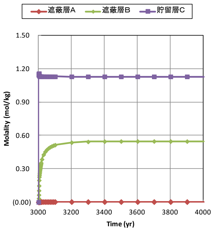
第 4.5-43 図 遮蔽層・貯留層境界付近での CO 2 飽和度と溶解 CO 2 量の時間変化（遮蔽性能（低）ケース）（平成 23 年度シミュレーション結果）
