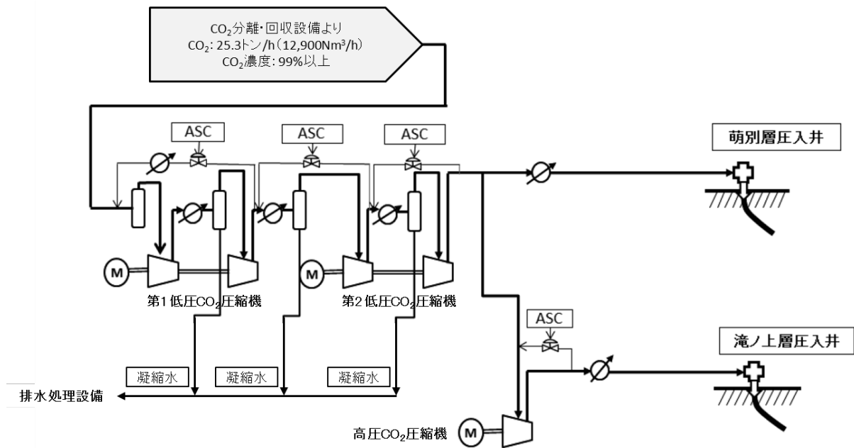
第 5.3-1 図 CO 2 圧縮設備構成
