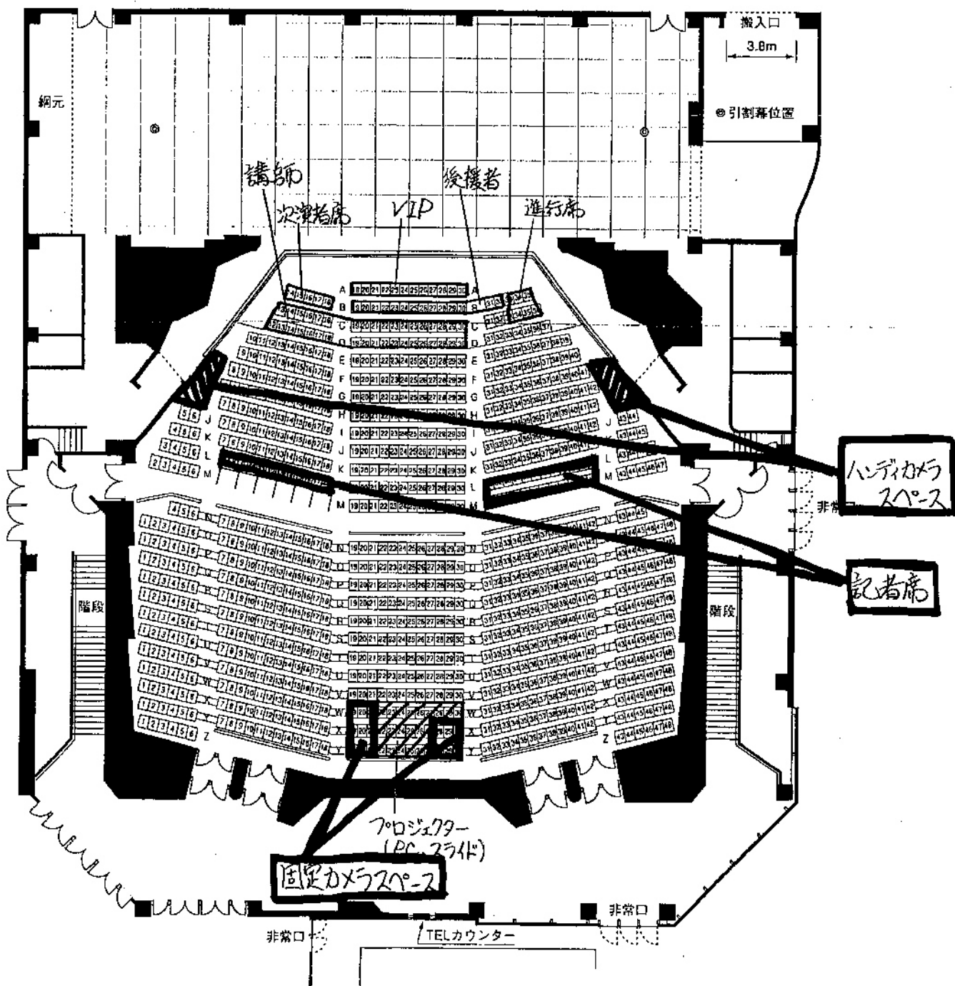
大ホール 平面図 (S : 1/200)
