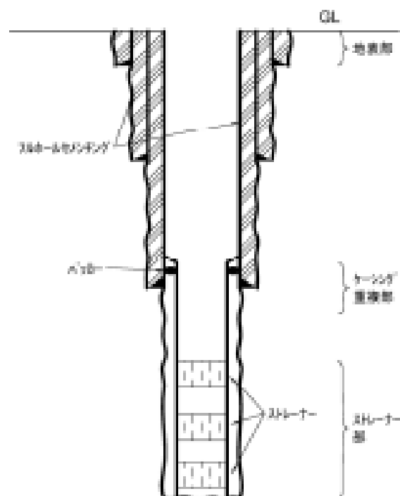
図 4 複径仕上げ井戸
