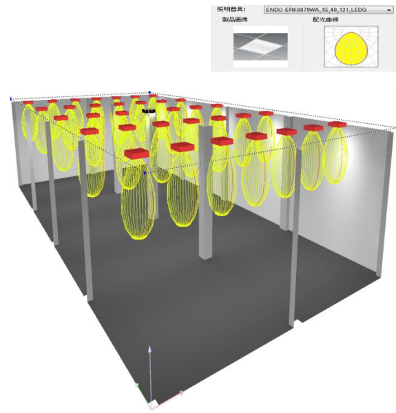
図2 配光の3D表示（例）
