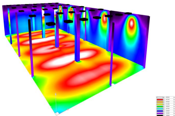
図3 計算結果一壁面及び床面の照度分布（例）
