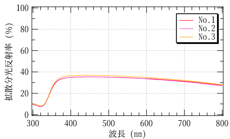
図-1 拡散分光反射率測定結果
