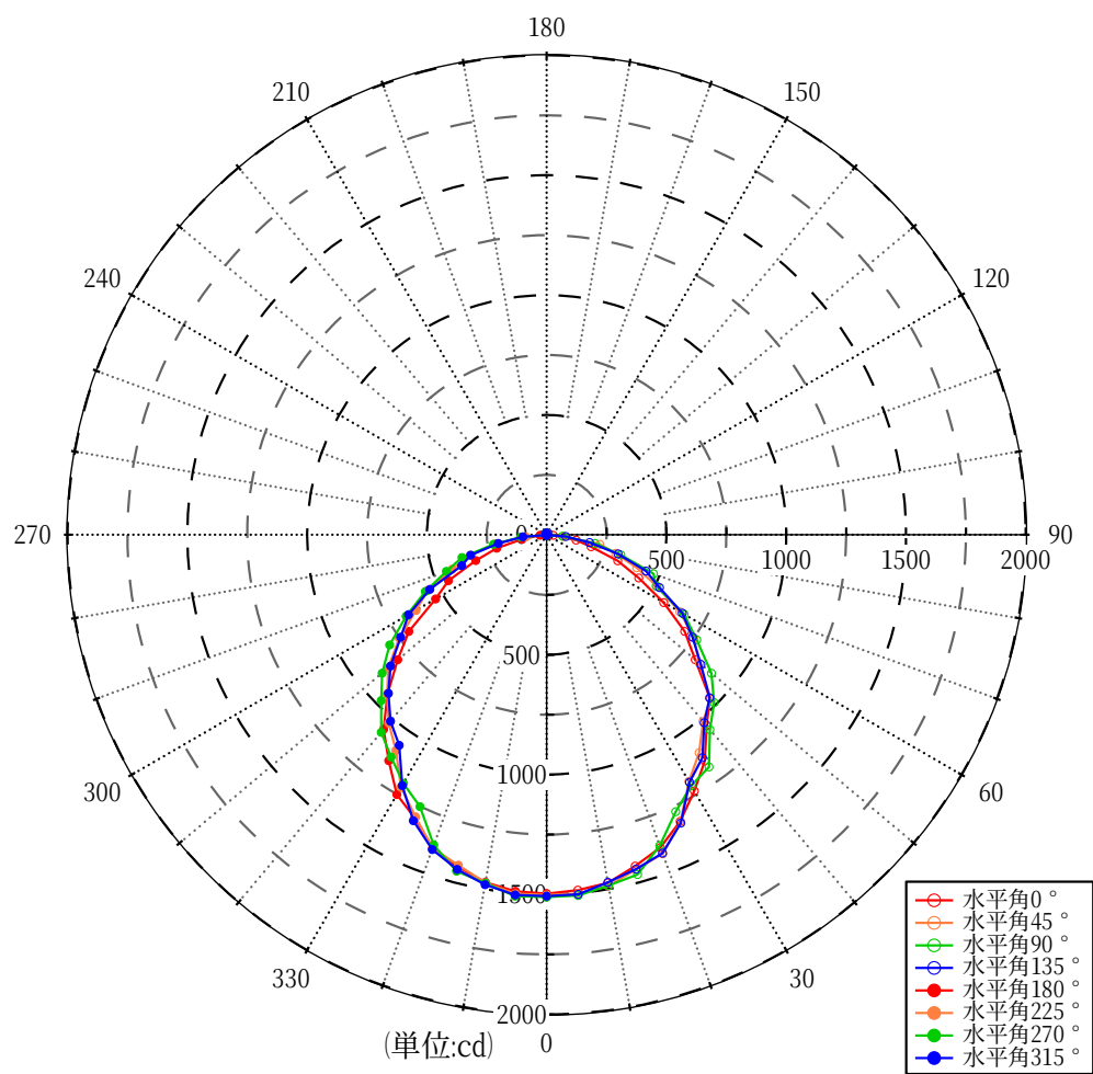
図-2 配光曲線
