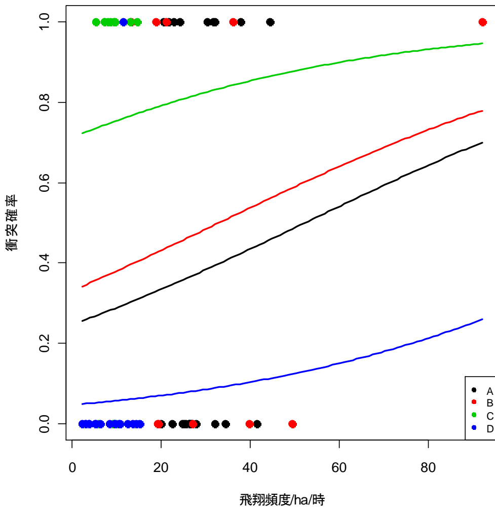
図 3-24 風車近傍における鳥類の飛翔頻度～衝突発生率(発生し易さ)
