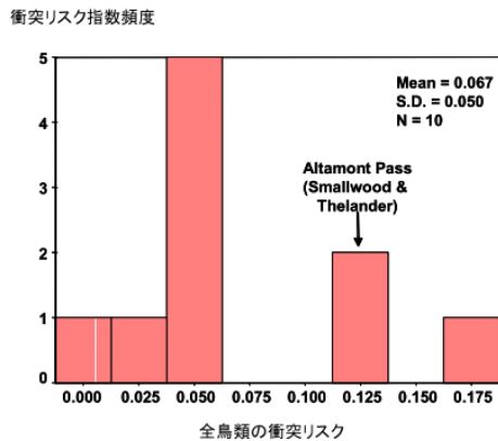
図 3- 19 Smallwood et al (2004)による飛翔頻度と衝突リスク
