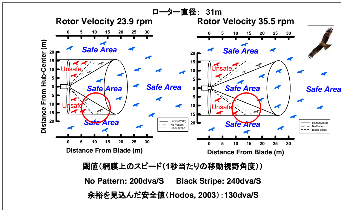
図 3-48 飛翔するトビからみた風車の視認性に関する模式図
