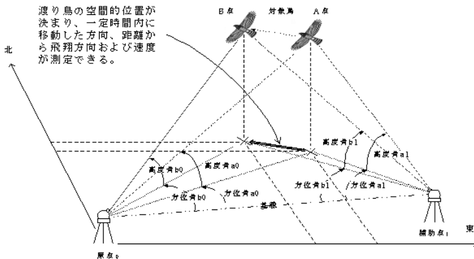
図3-29 セオドライトによる鳥類の飛翔経路測定
