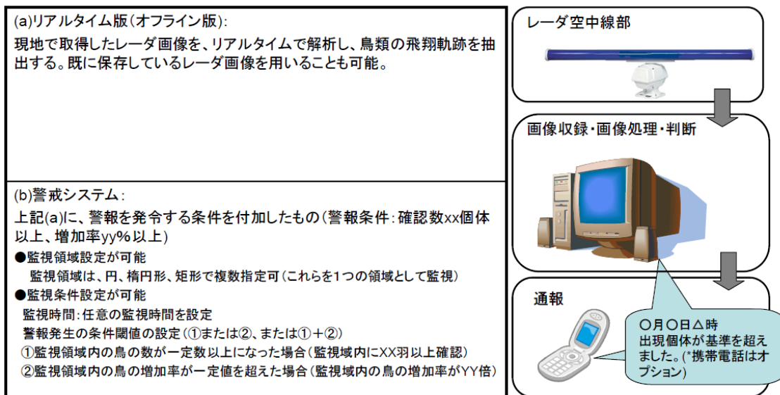
図 3- 53 システム構成
