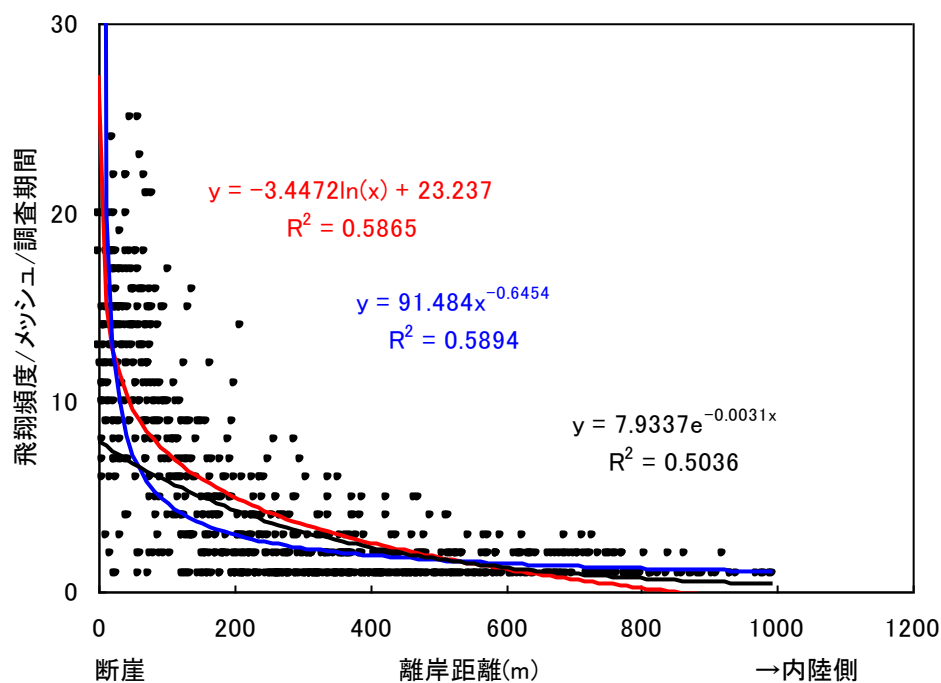
図 3- 25 環境勾配(離岸距離)と飛行頻度の関係
