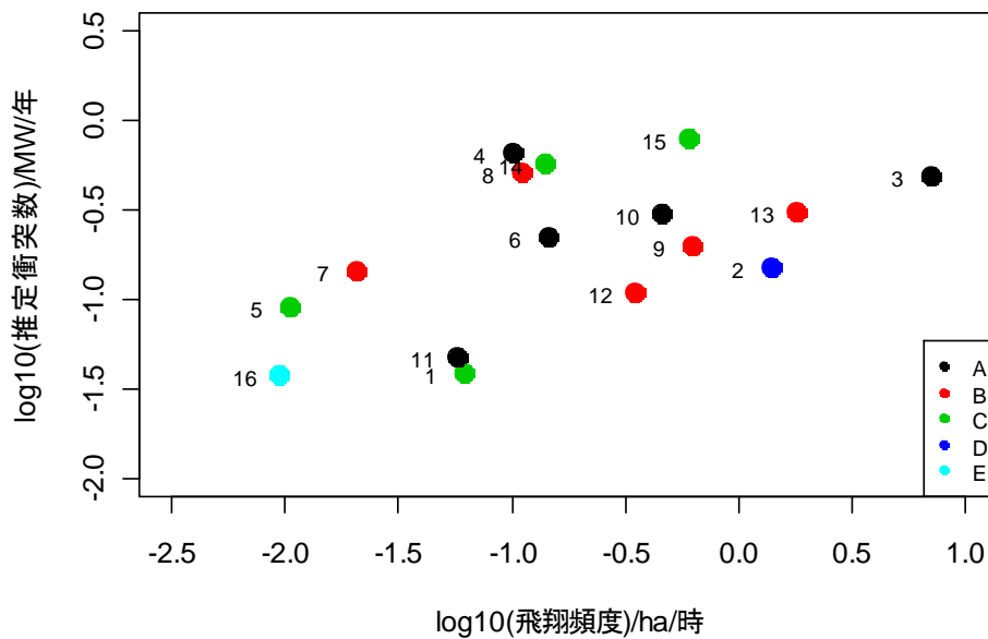
図 3-21 風車近傍における鳥類種別飛行頻度～推定衝突数
