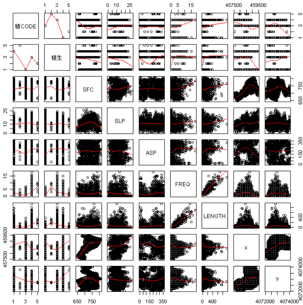
図 3-36 散布図行列の例
