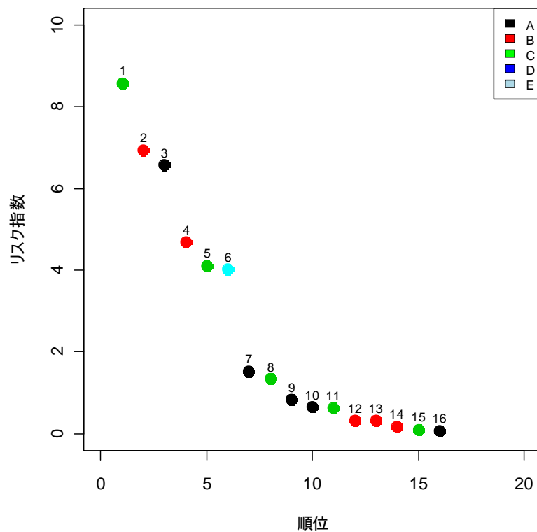
図 3-59 衝突リスク指数(鳥類種別、風力発電施設別)
