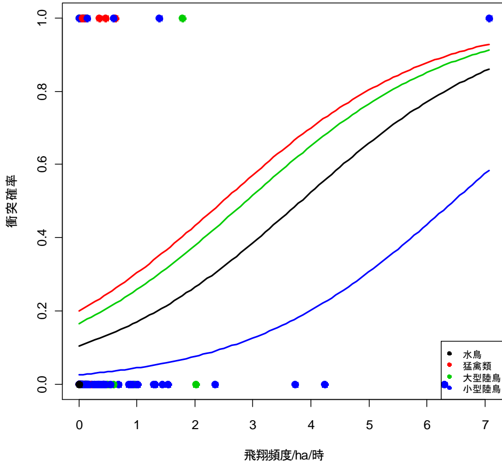
図 3- 23 分類群別にみた飛行頻度～衝突発生率(発生し易さ)
