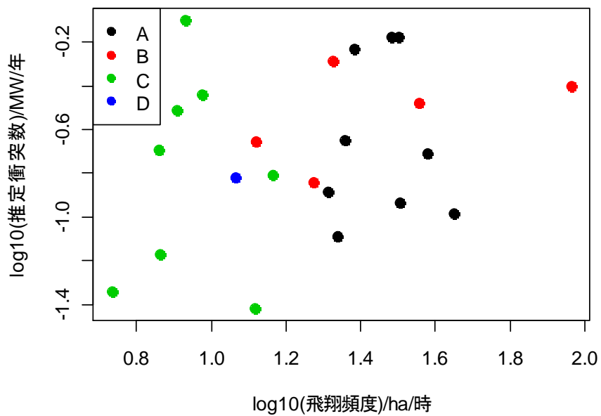
図 3-22 風車近傍における鳥類の飛行頻度～推定衝突数
