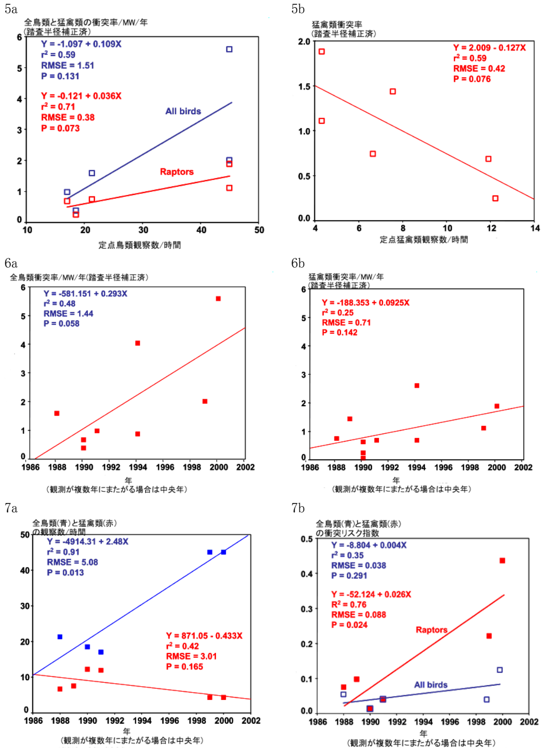
図 3-20 Smallwood et al (2004)による飛翔頻度と衝突リスク(つづき)
