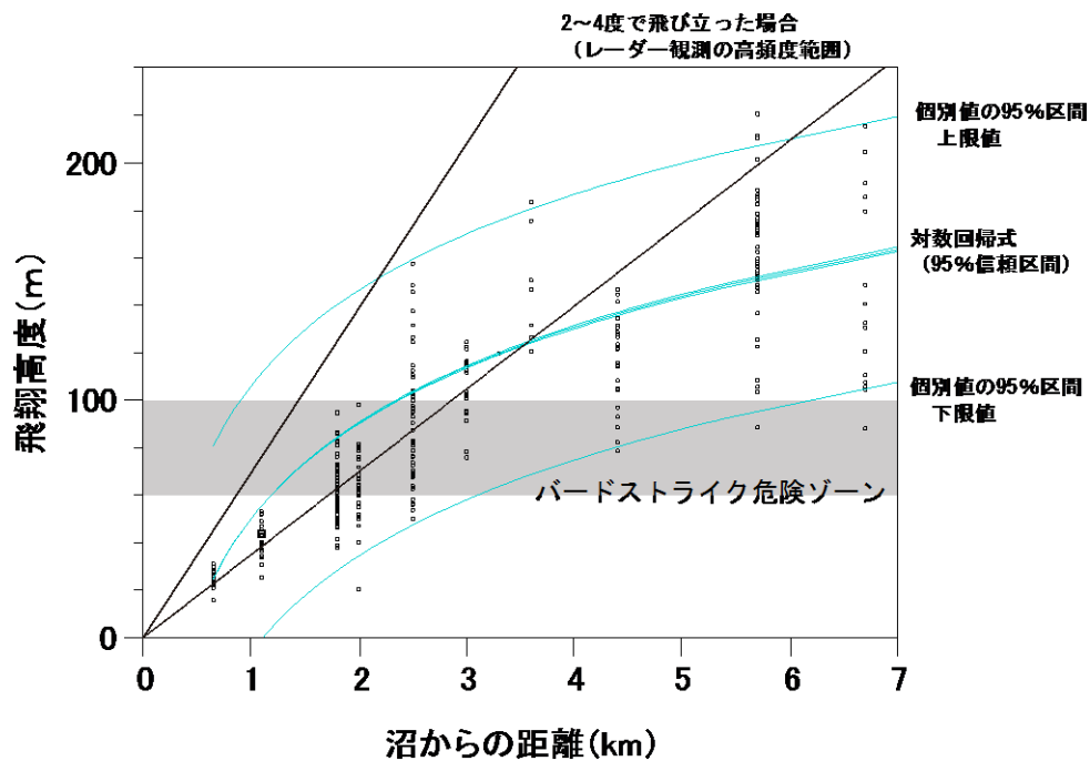
図 3-17 渡りおよび長距離移動するマガンの飛翔高度と飛び立ち地点からの距離との関係。 ●が風の強かった日の記録、+がそれ以外の日の記録。実線は対数回帰式による推定で破線は 95%信頼区間。 網掛けした高度はバードストライクの危険のある高度。
