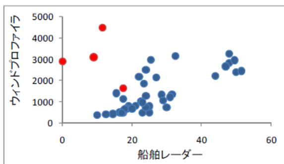
図 3- 32 ウィンドプロファイラと船舶レーダの渡り鳥エコー頻度の比較(1 時間値: 環境省 2008d)
