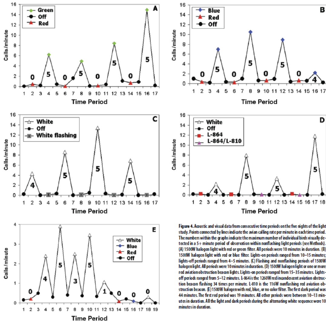
図 3- 51 照明実験による夜間に渡る鳥類(鳴き声の確認数)の変化 (Evans et al 2007 より抜粋)
