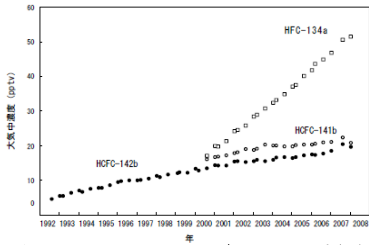
図5 北海道における HCFC-141b、HCFC-142b 及び HFC-134a の大気中平均濃度の経年変化
