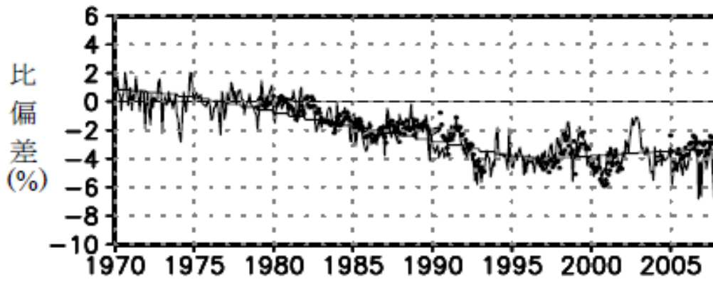
図1 世界のオゾン全量の変化の度合い 気象庁 オゾン層観測報告 2007 より
