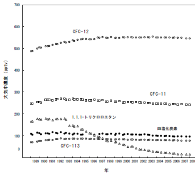
図3 北海道におけるCFC等の大気中平均濃度の経年変化
