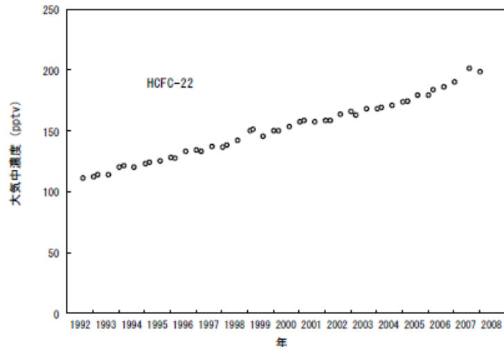
図4 北海道における HCFC-22 の大気中平均濃度の経年変化
