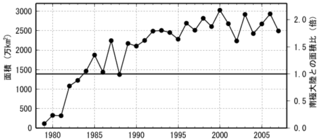
図2 オゾンホール面積の経年変化 気象庁 オゾン層観測報告 2007 より
