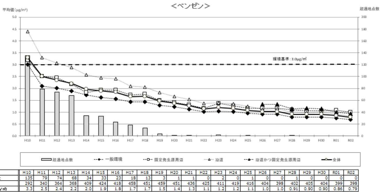
図2 平均值及び環境基準超過地点数の推移（環境基準が設定されている物質）
