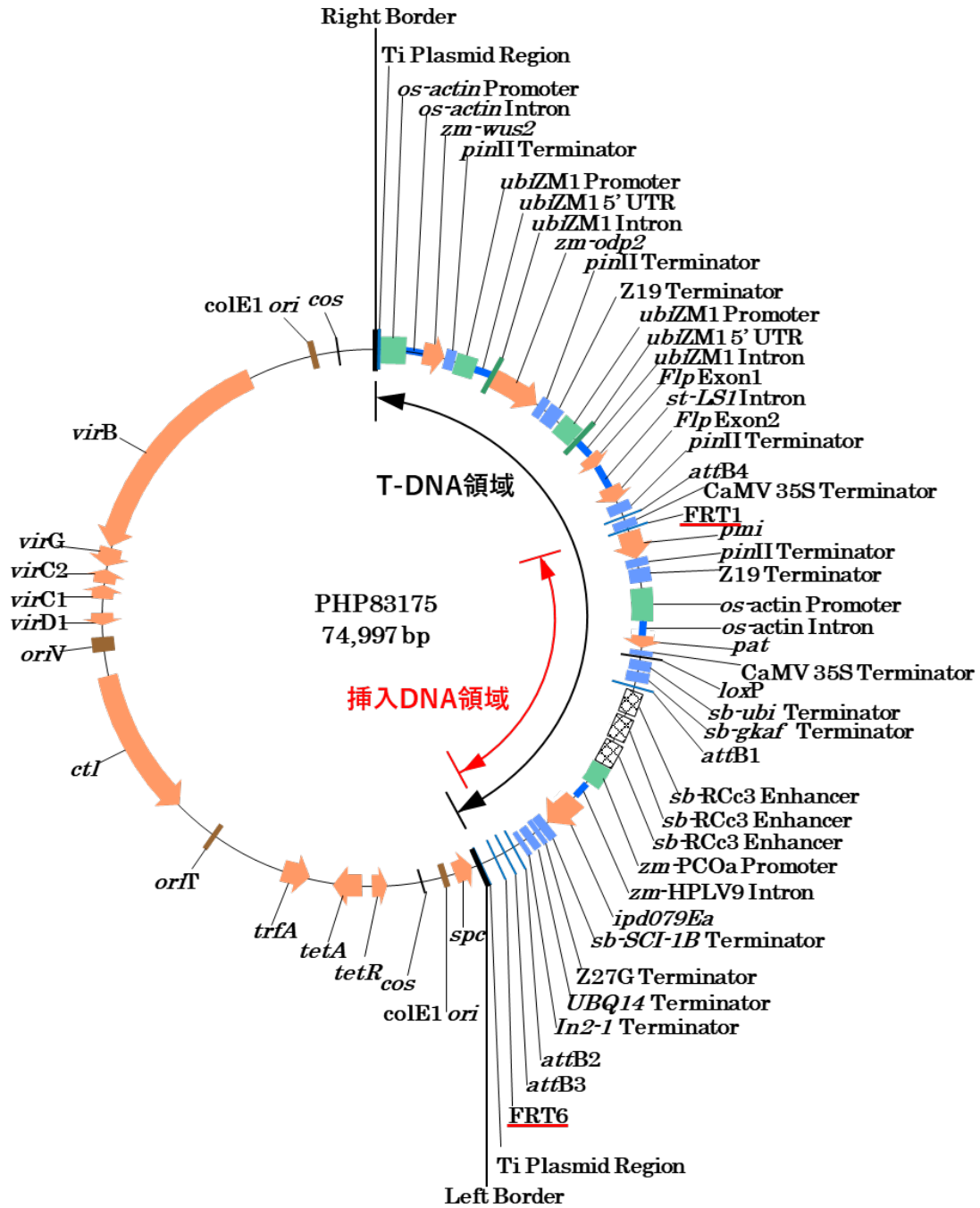
図 3 プラスミド PHP83175 における供与核酸の構成 染色体に挿入される領域は、赤下線で示した FRT1 及び FRT6 に挟まれた挿入 DNA 領域である。
