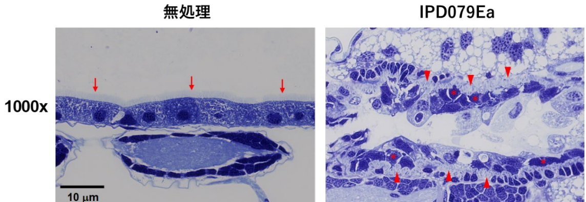
図 2 IPD079Ea 投与後の WCR 中腸
