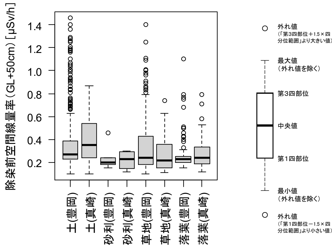
除染場所の空間線量率(事前測定:2013年9月～11月)
