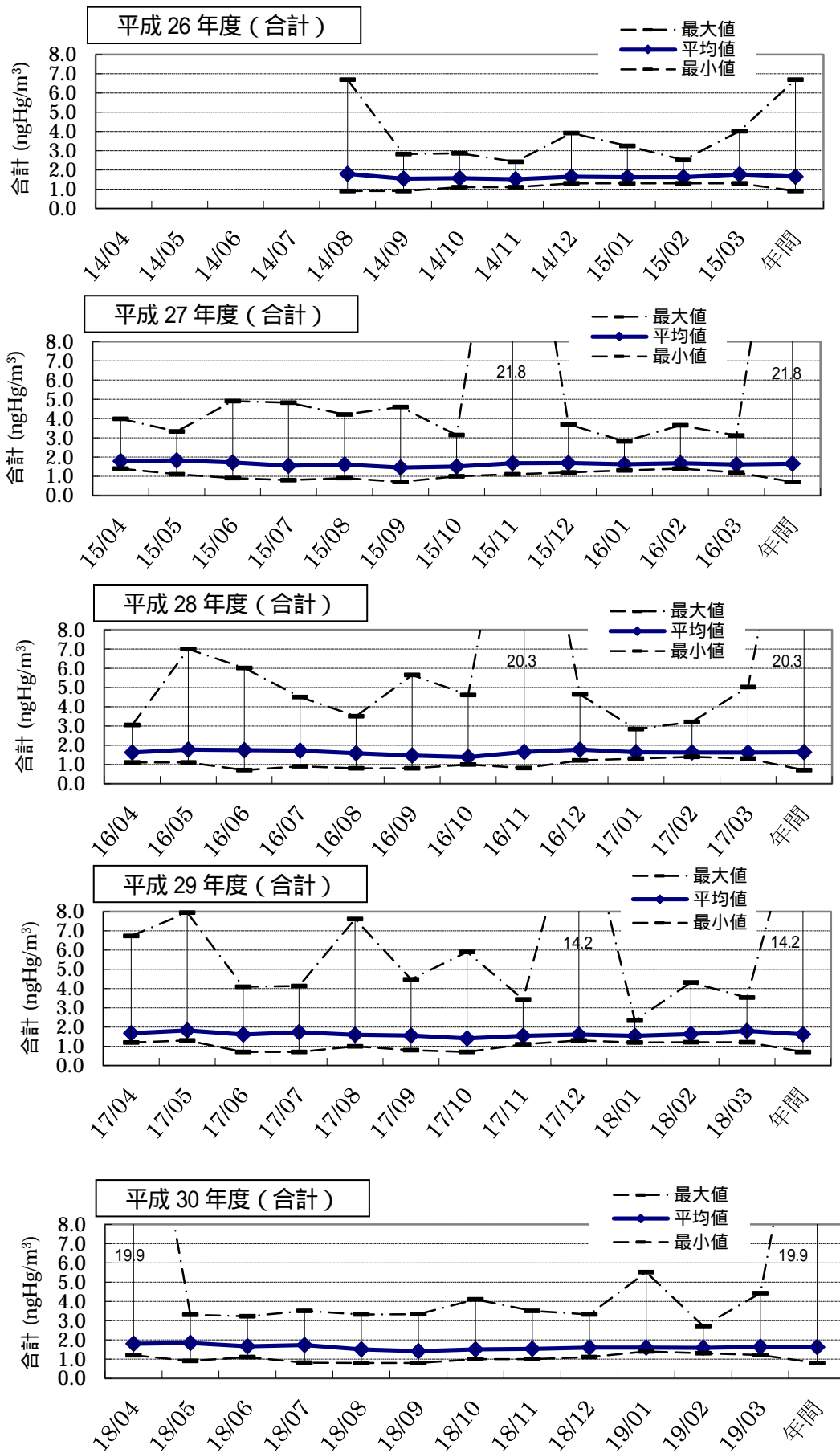
図5 男鹿半島における大気中水銀濃度の推移(月別平均値、範囲)
