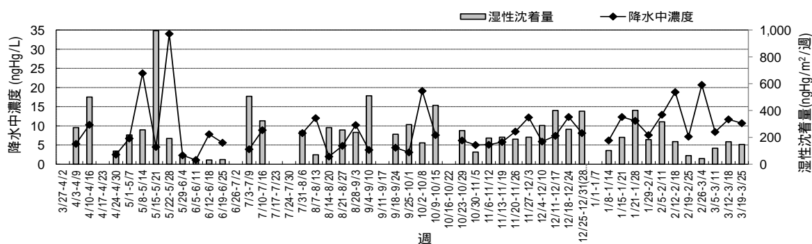
図 8 男鹿半島における降水中水銀濃度及び湿性沈着量 (平成 30 年度)
