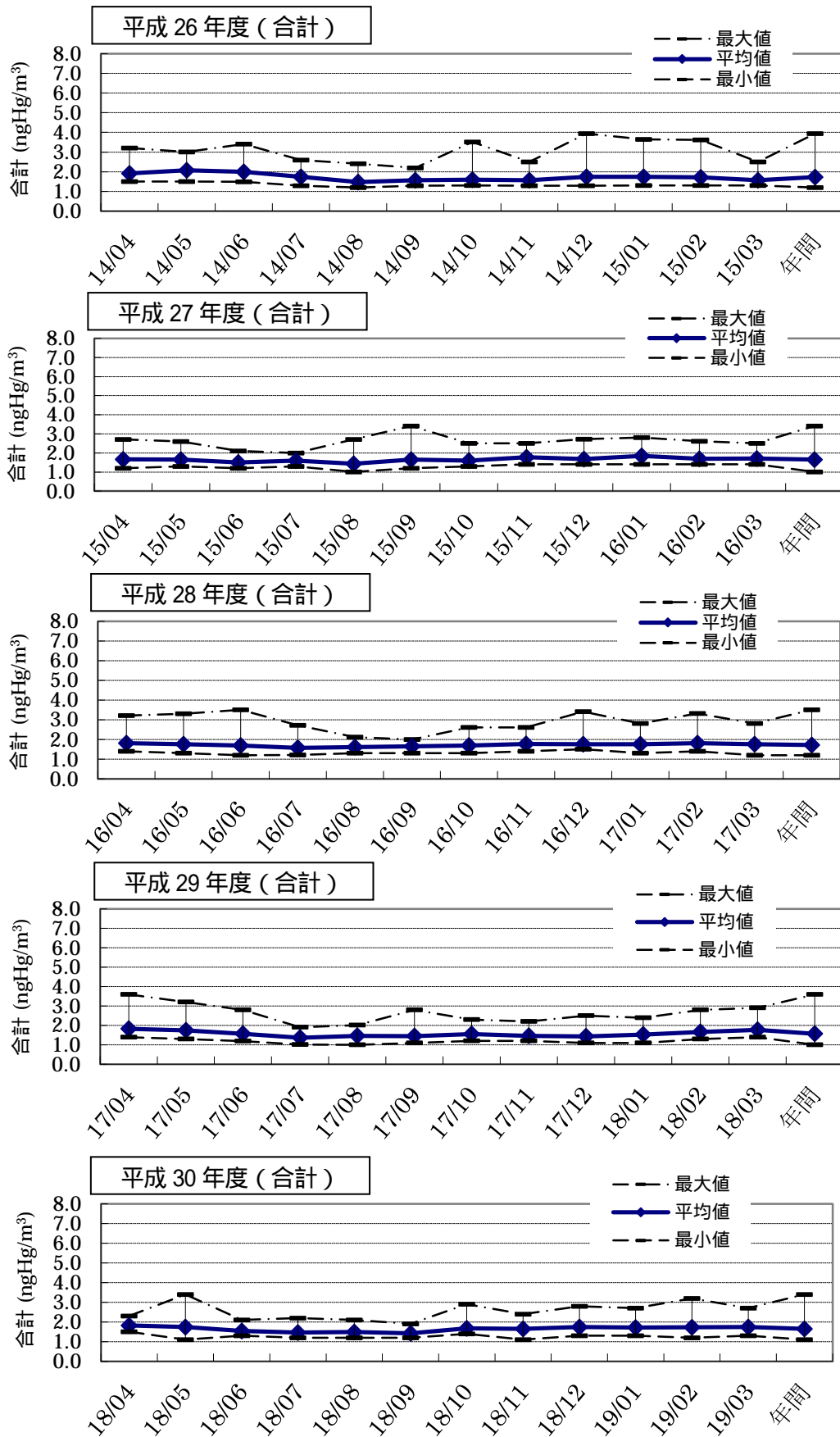
図 3(2) 辺戸岬における大気中水銀濃度の推移(月別平均値、範囲)
