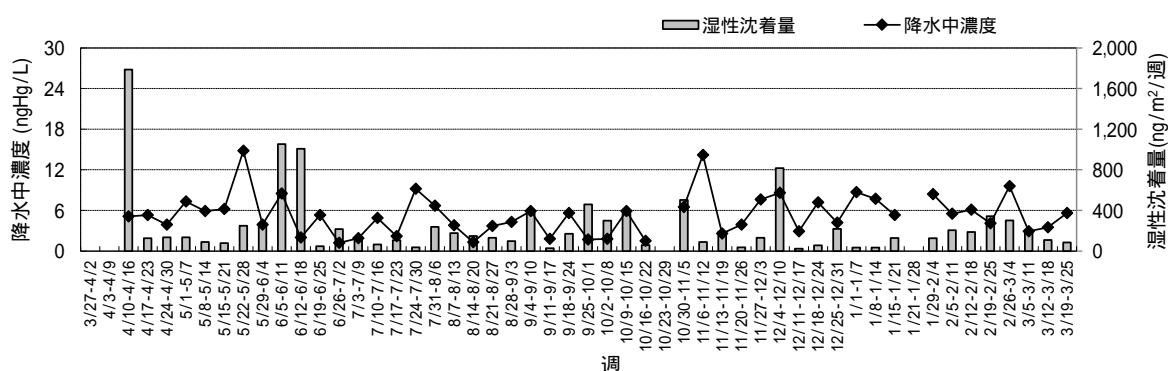
図 6 辺戸岬における降水中水銀濃度及び湿性沈着量(平成 30 年度)
