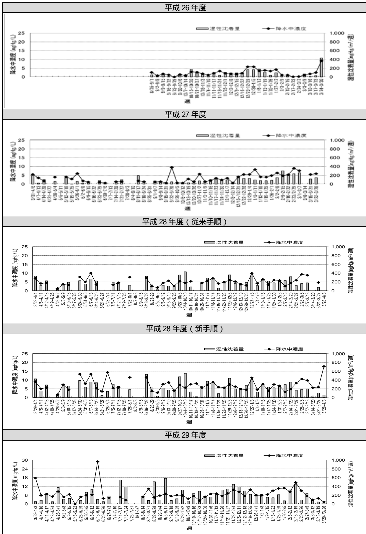
図9 男鹿半島における降水中水銀濃度及び湿性沈着量の推移
