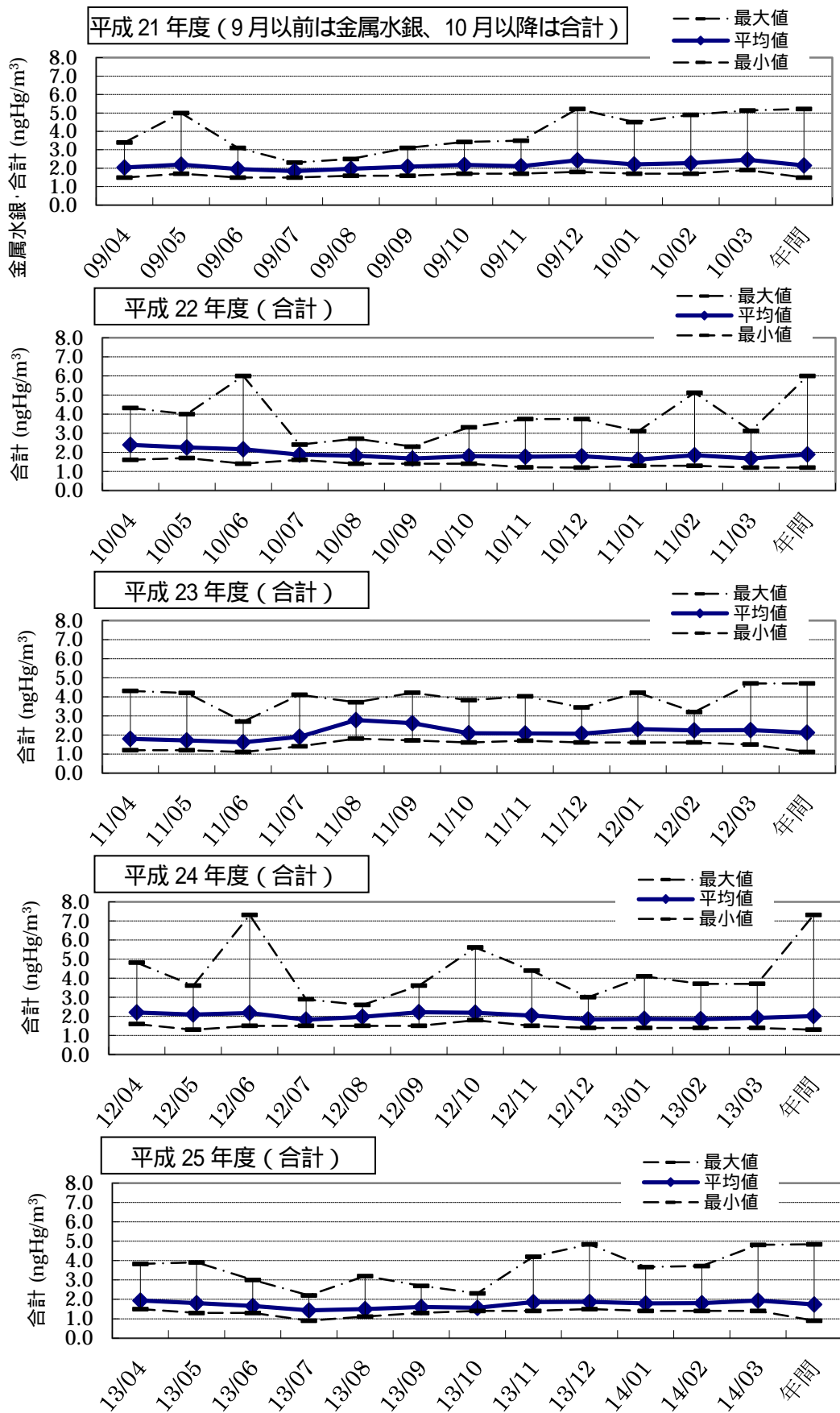
図 3(1) 辺戸岬における大気中水銀濃度の推移(月別平均値、範囲)
