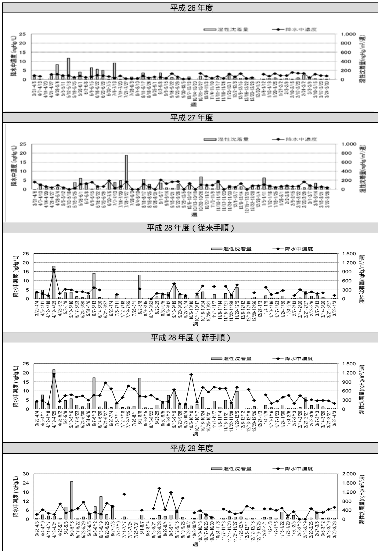
図 7(2) 辺戸岬における降水中水銀濃度及び湿性沈着量の推移
