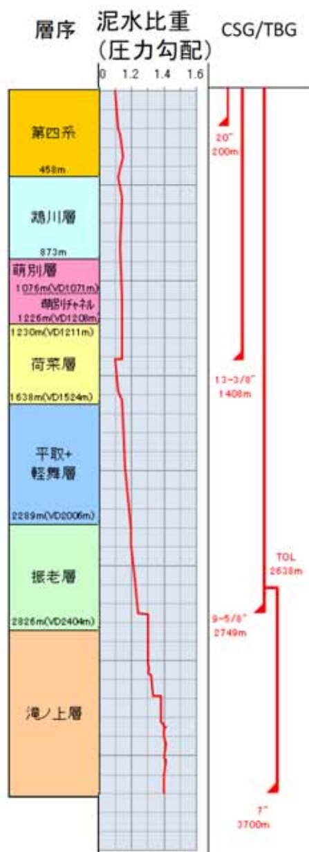
図 2.2-4 苦小牧 CCS-1 における泥水比重の変化図
