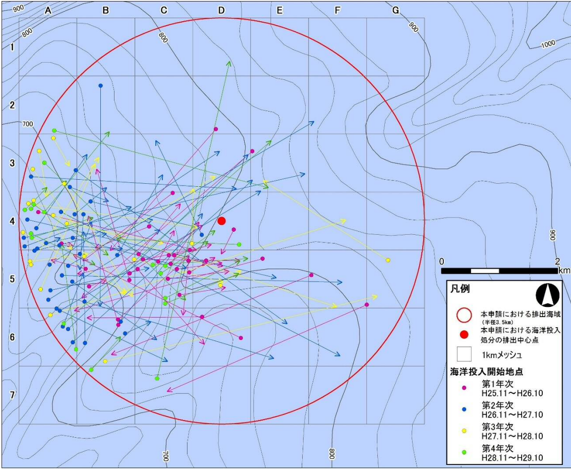
図面-3 (廃棄物投入範囲図)
