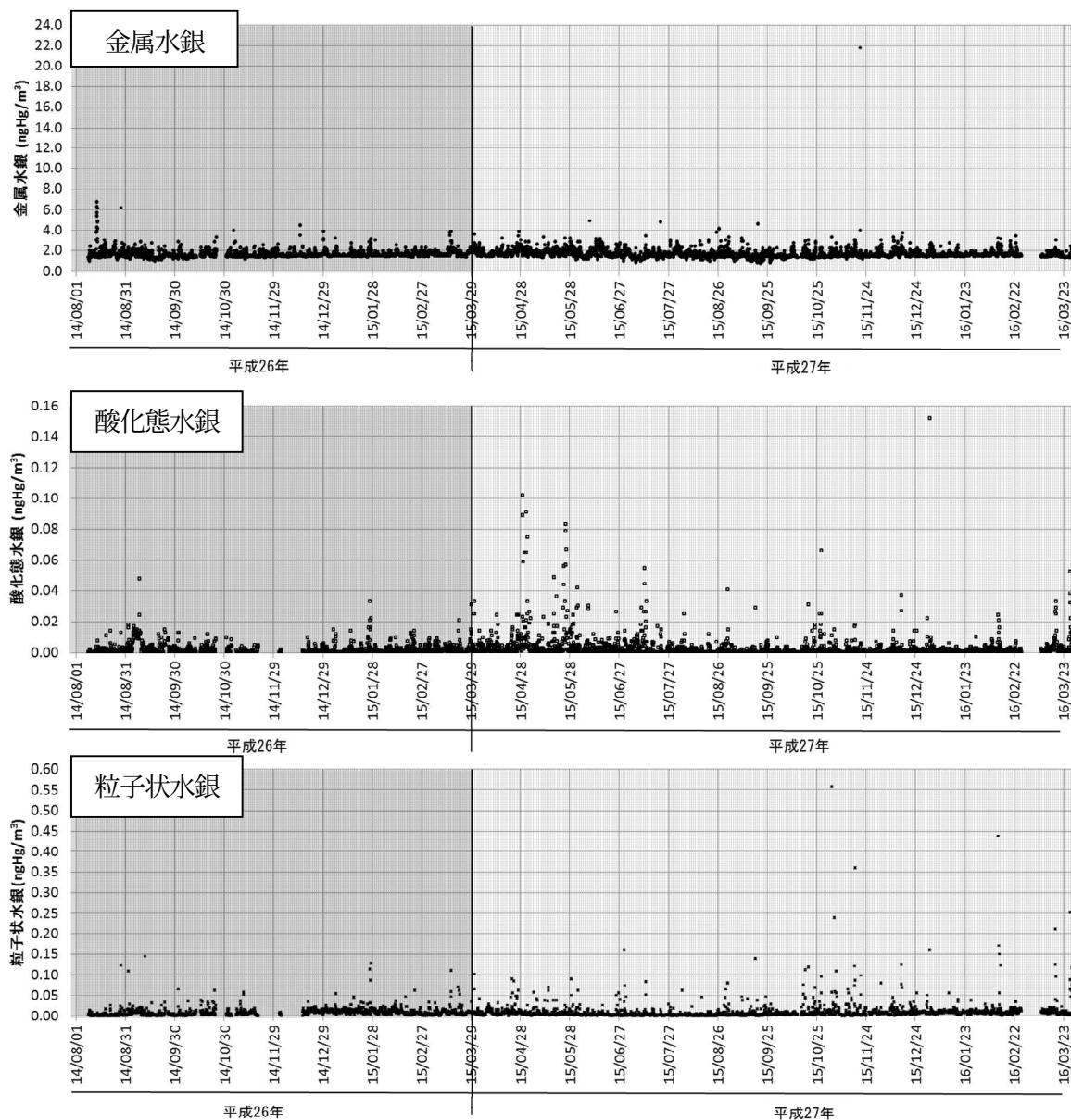
図 7 男鹿における大気中形態別水銀濃度の測定結果の経年変化
