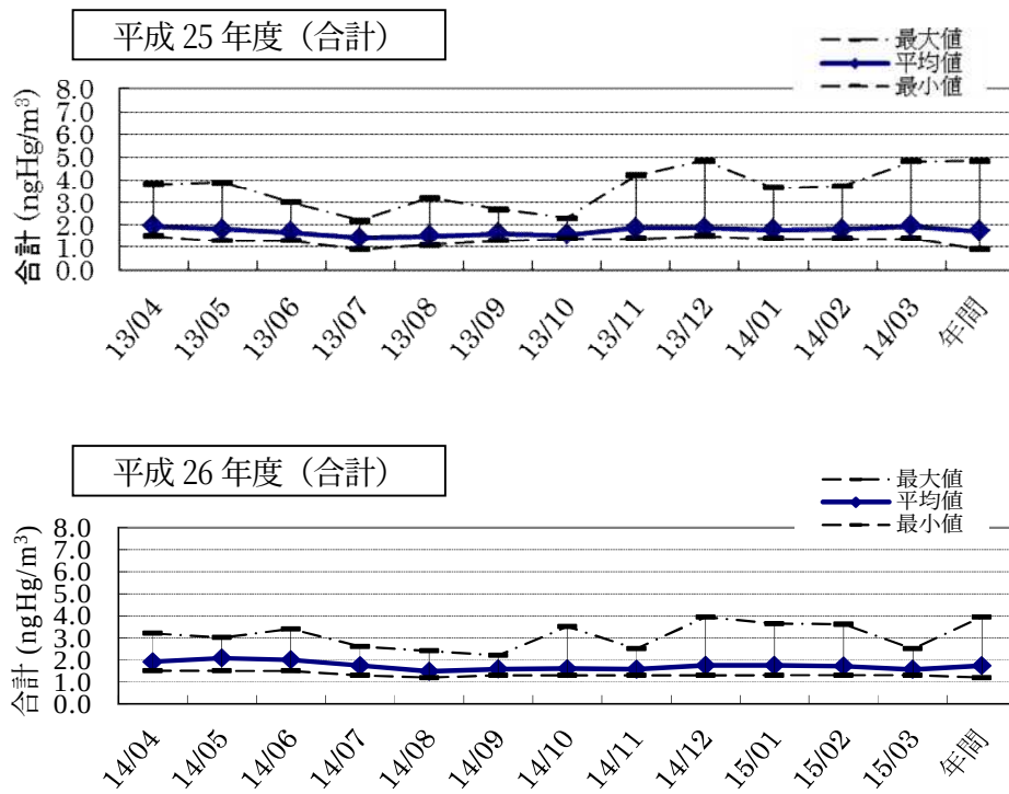
図 4(2) 辺戸岬における大気中水銀濃度の過年度調査結果(月別平均値、範囲)
