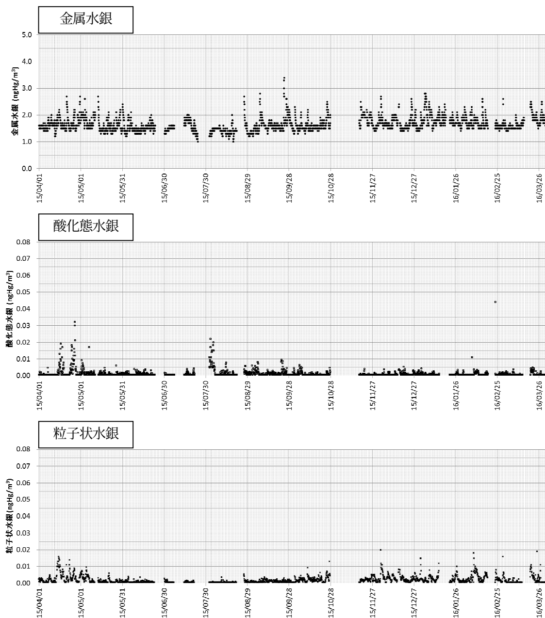
図1 辺戸岬における大気中形態別水銀濃度の測定結果（平成 27 年度）
