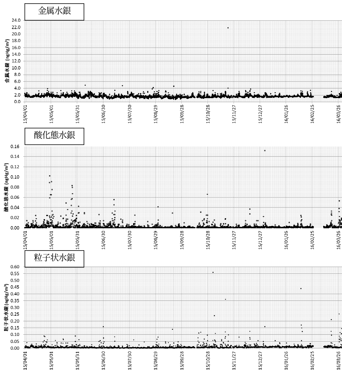
図5 男鹿半島における大気中形態別水銀濃度の測定結果（平成 27 年度）
