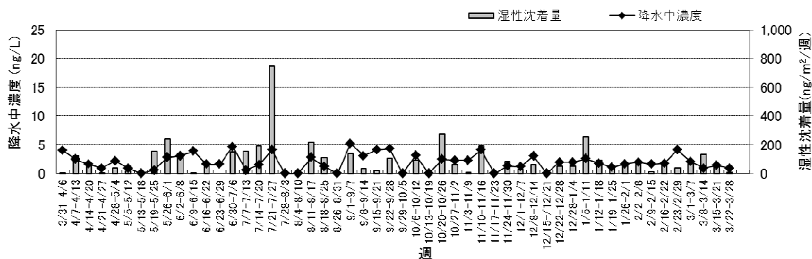
図 9 辺戸岬における降水中水銀濃度及び湿性沈着量（平成 27 年度）
