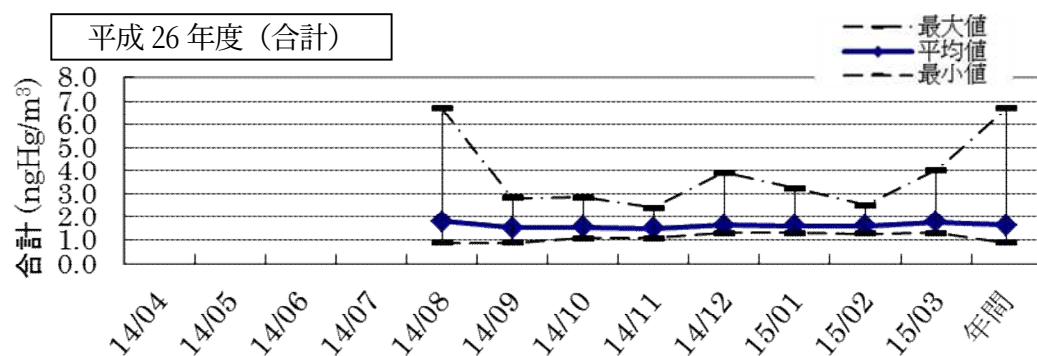
図8 男鹿における大気中水銀濃度の過年度調査結果(月別平均値、範囲)
