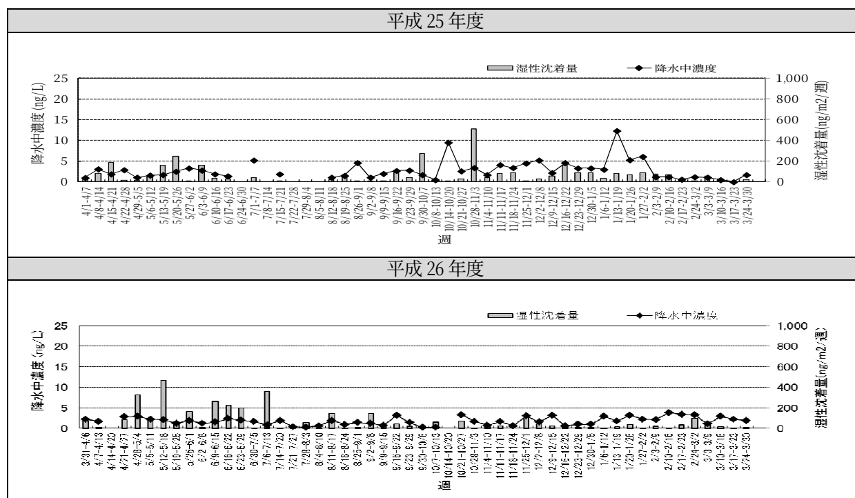
図 10(2) 辺戸岬における降水中水銀濃度及び湿性沈着量の過年度調査結果
