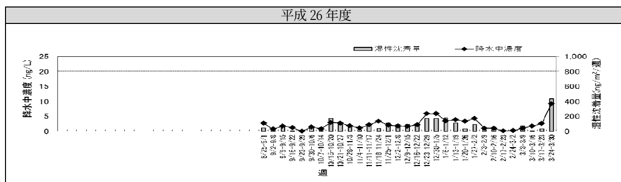
図 12 男鹿における降水中水銀濃度及び湿性沈着量の過年度調査結果
