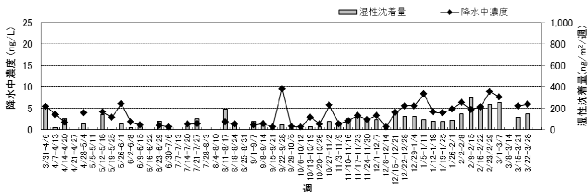
図 11 男鹿半島における降水中水銀濃度及び湿性沈着量 (平成 27 年度)
