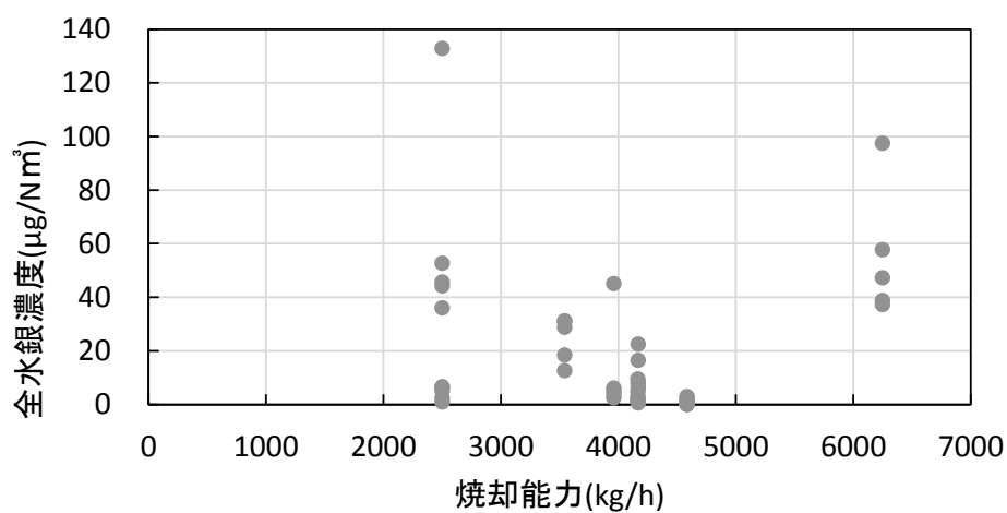
図Ⅱ-4-2-6 焼却能力と全水銀濃度との関係
