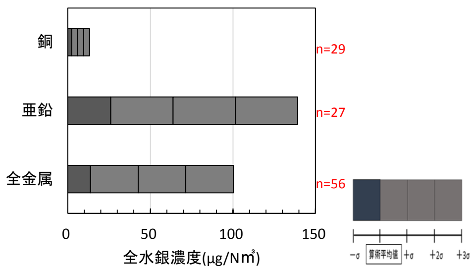
図Ⅱ-2-8 一次施設の金属種類と濃度分布（環境省法以外）
