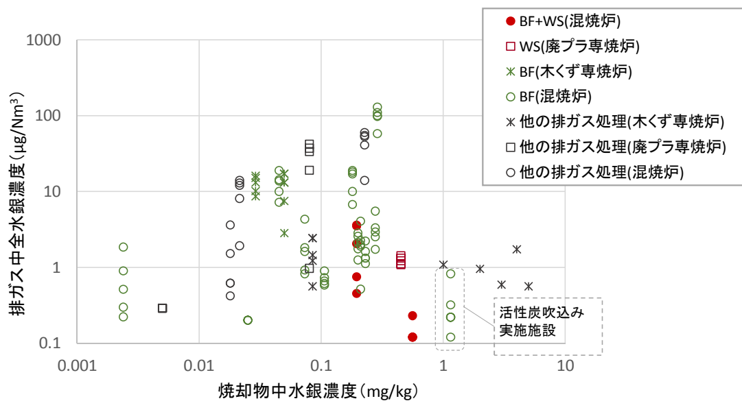
図Ⅱ-4-1-9 排ガス処理設備ごとの焼却物中水銀濃度と全水銀濃度 (産業廃棄物焼却炉)
