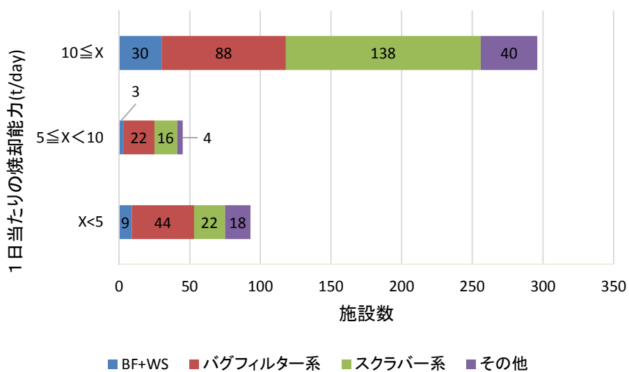
図Ⅱ-4-1-2 施設規模・集じん機別の炉数（全国、使用開始年 1995 年以前）
