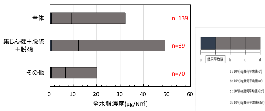
図Ⅱ-1-10 排ガス処理設備の種類ごとの全水銀濃度 (対数標準偏差)
