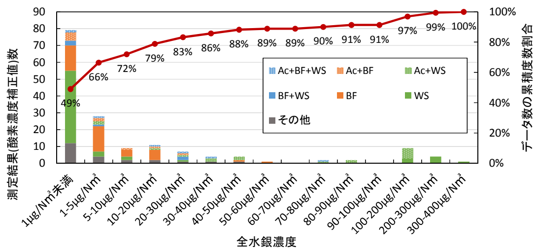
図Ⅱ-4-1-17 排ガス中水銀濃度ヒストグラム（産業廃棄物焼却炉）（環境省法以外）
