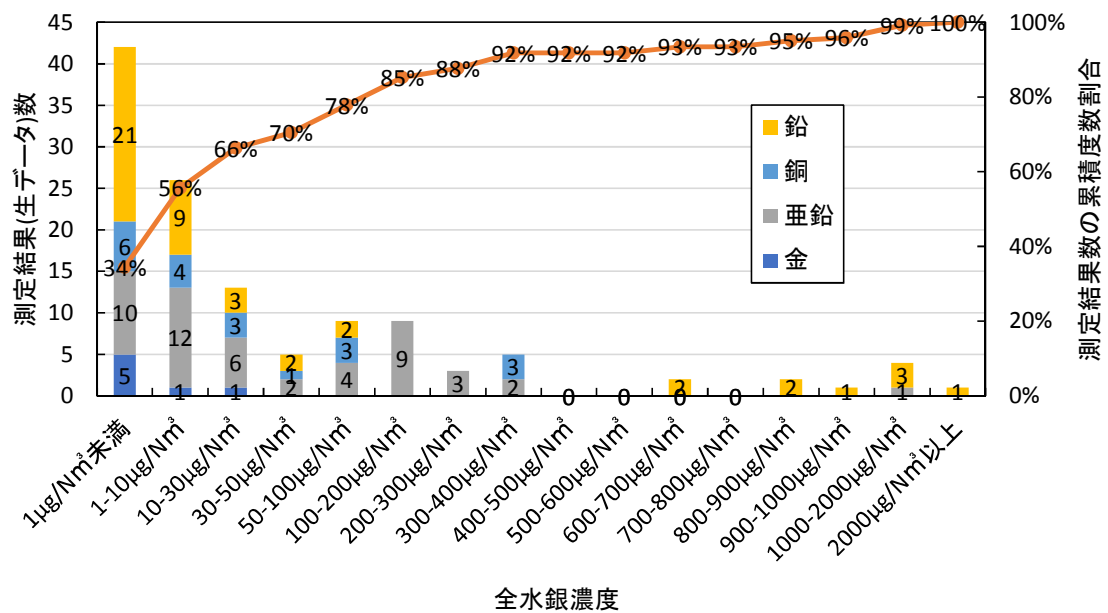
図 II-3-4 二次施設における金属種類と排ガス中全水銀濃度
