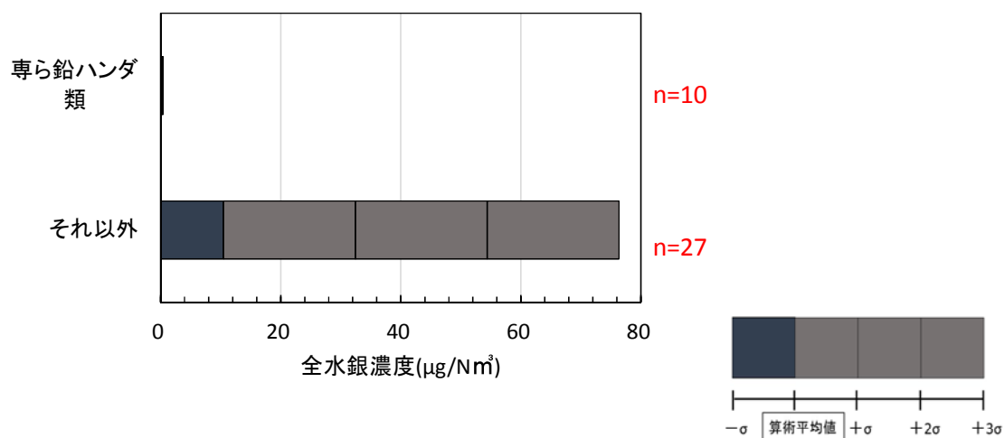
図Ⅱ-3-7 鉛二次施設における原料の種類と全水銀濃度
