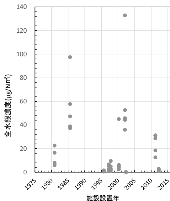
図Ⅱ-4-2-5 施設設置年と全水銀濃度との関係
