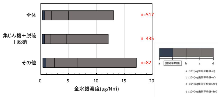
図Ⅱ-1-25 排ガス処理設備の種類ごとの水銀濃度（対数標準偏差） （小型石炭混焼ボイラー以外）（環境省法以外）
