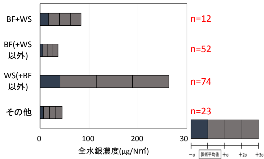
図Ⅱ-4-1-18 排ガス処理方式と全水銀濃度（産業廃棄物焼却炉）（環境省法以外）
