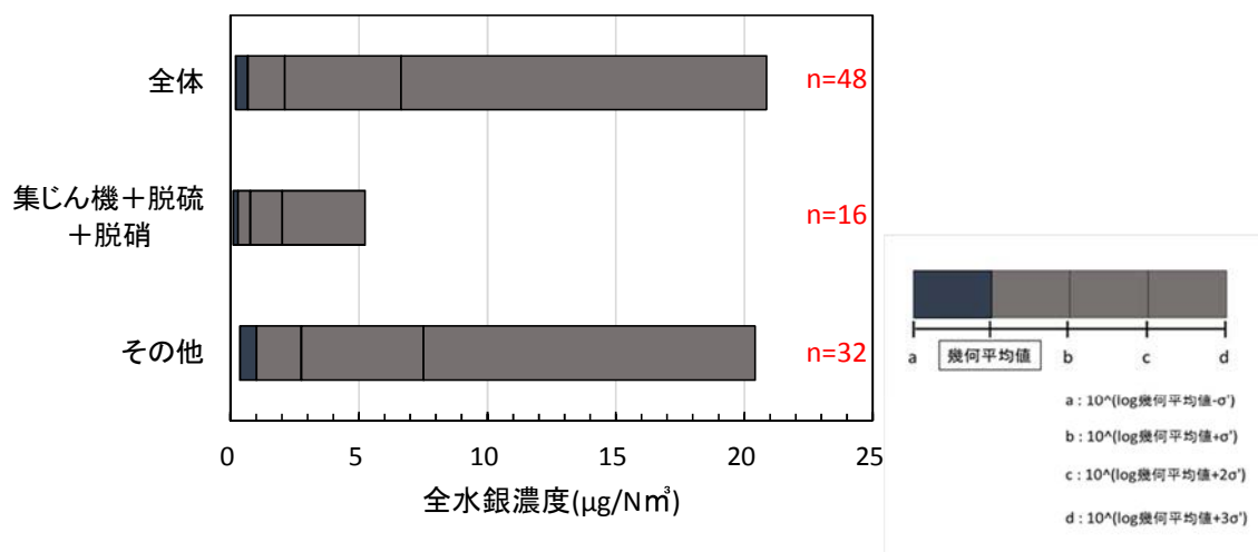
図Ⅱ-1-22 排ガス処理設備の種類ごとの水銀濃度（対数標準偏差） （小型石炭混焼ボイラー）（環境省法以外）
