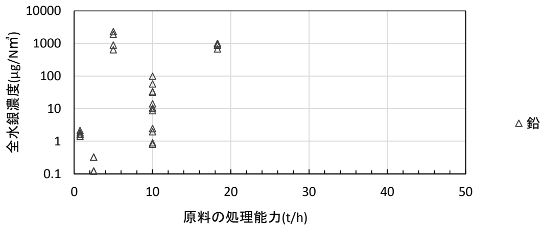
図Ⅱ-3-9 処理能力と全水銀濃度との関係（鉛二次施設）
