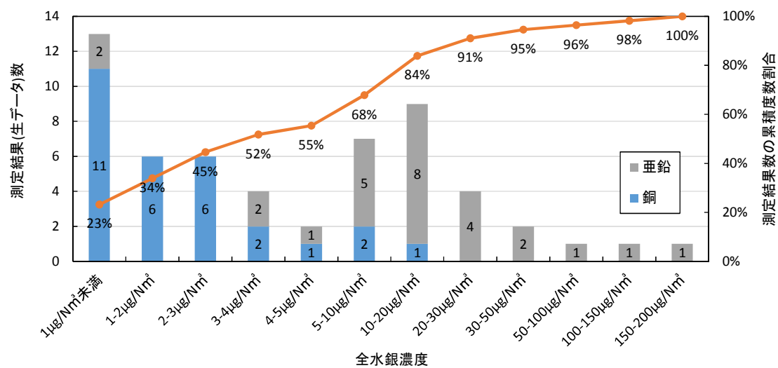
図Ⅱ-2-7 一次施設における金属種類と水銀濃度（環境省法以外）
