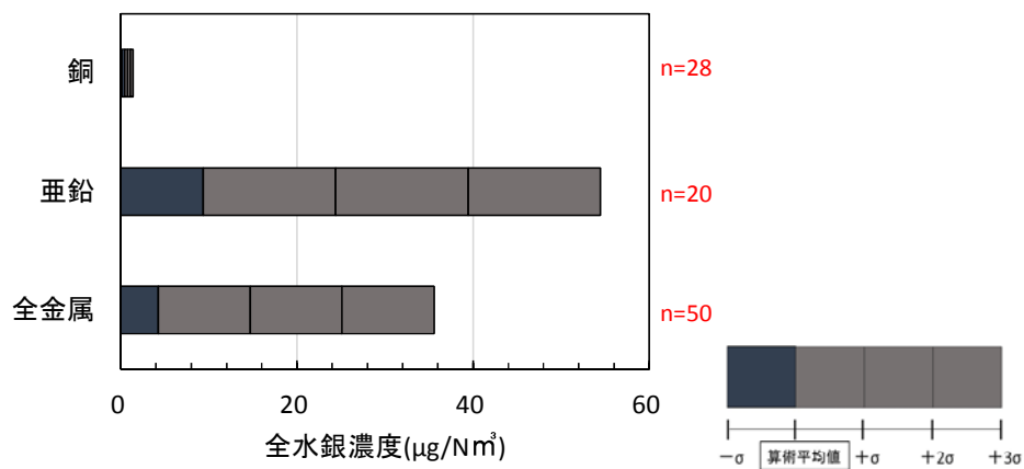
図 II-2-5 一次施設の金属種類と濃度分布
