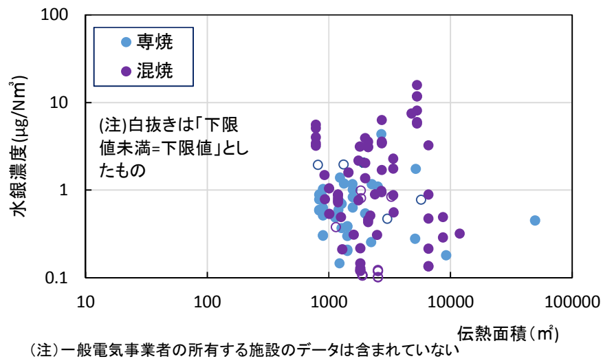
図 II-1-6 伝熱面積と全水銀濃度
