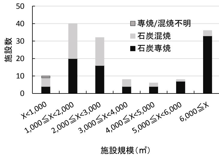
図Ⅱ-1-1 伝熱面積による規模分布
