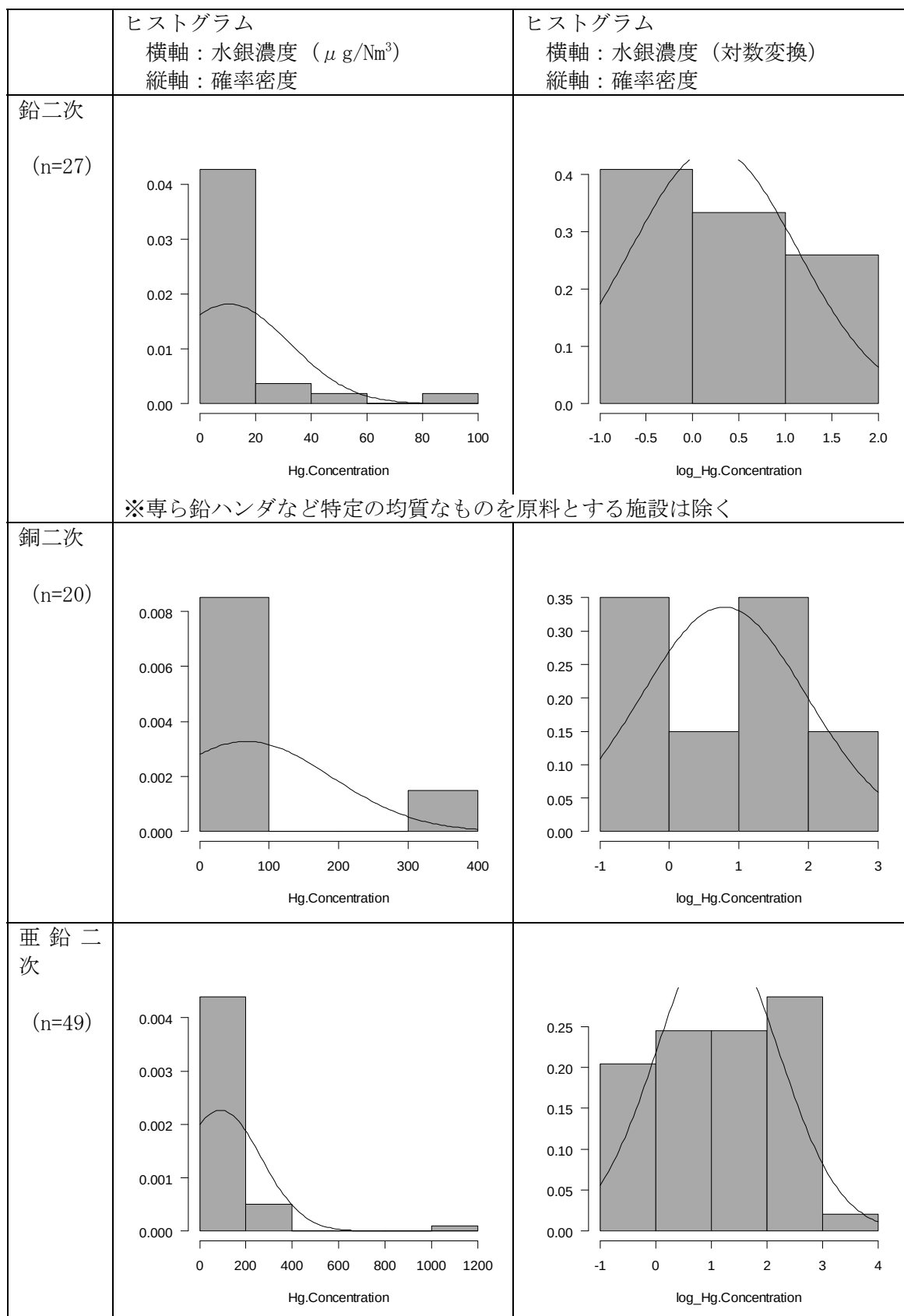
図Ⅲ-5-3 排ガス中の水銀濃度（全水銀）のヒストグラム（非鉄二次施設）（1/2）
