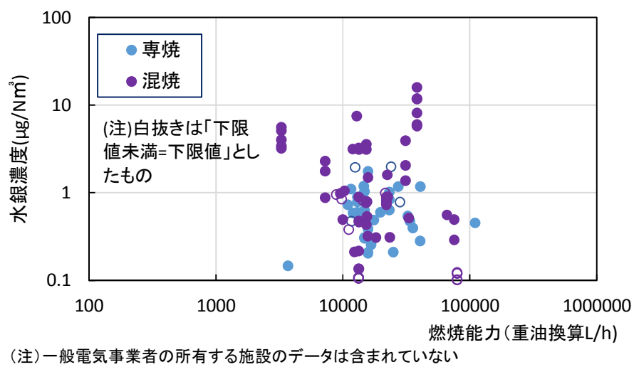
図 II-1-7 燃焼能力と全水銀濃度
