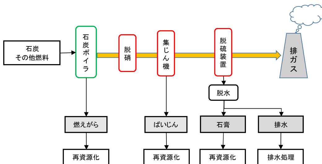
図Ⅱ-1-4 石炭火力発電所及び産業用石炭燃焼ボイラーの排ガス処理設備
