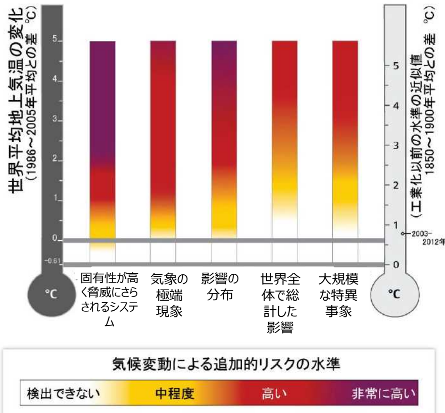
図. 気温上昇と、それに伴うリスク上昇 (出所) AR5 WG2 SPM Assessment Box SPM.1 図.1
