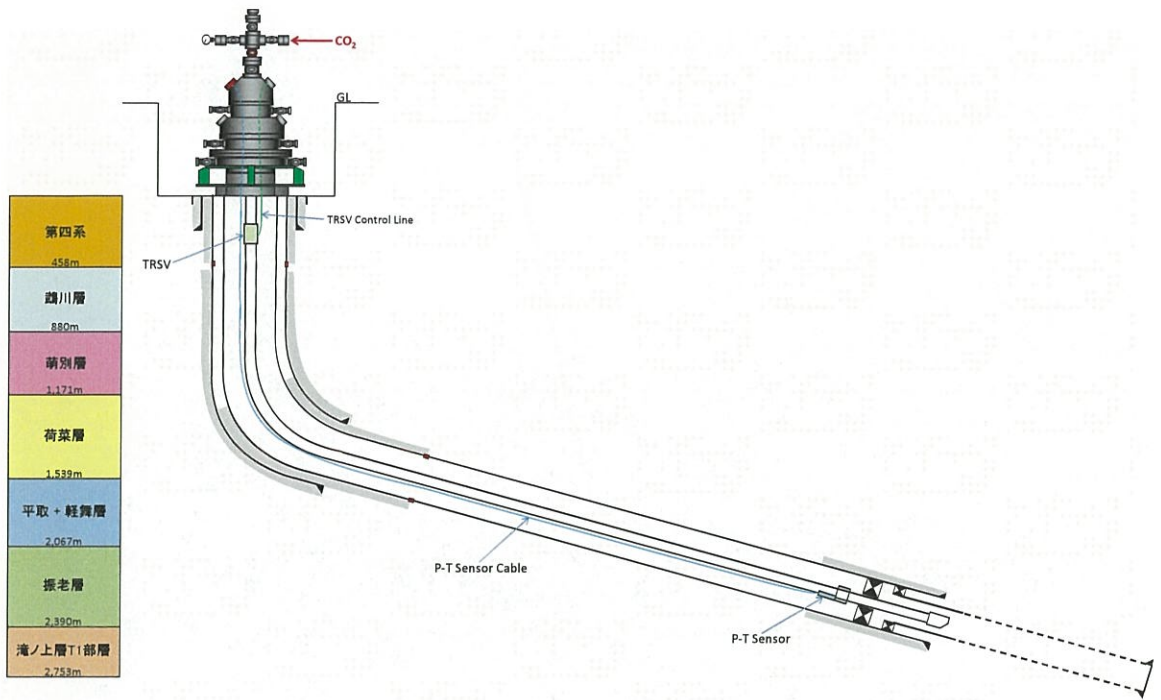
第 5. 3-2 図 滝ノ上層圧入井の概要
