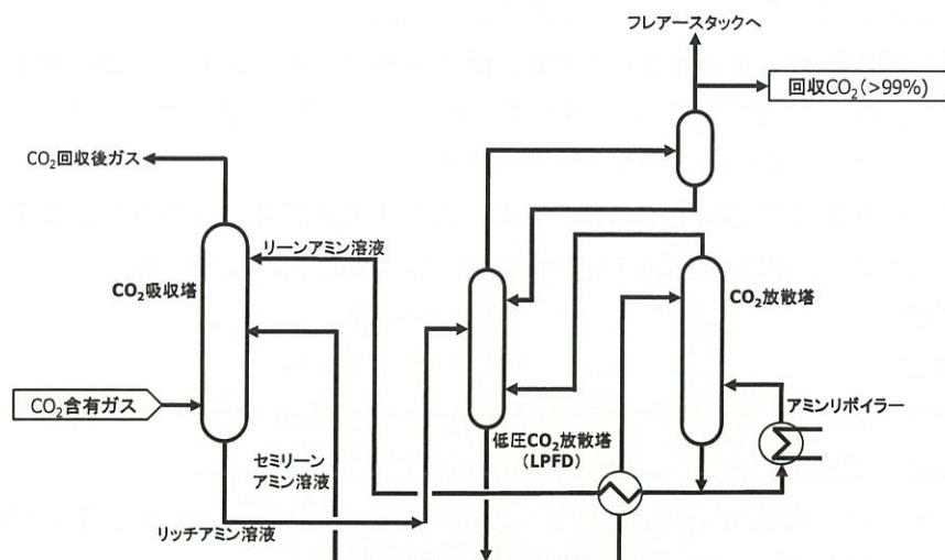
第 5. 1-1 図 CO 2 分離・回収設備構成
