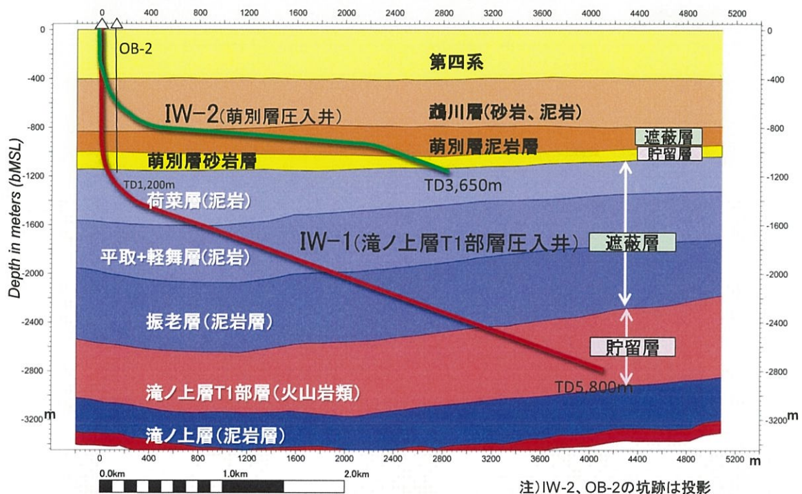
第 1.3-1 図 苫小牧地点の層序
