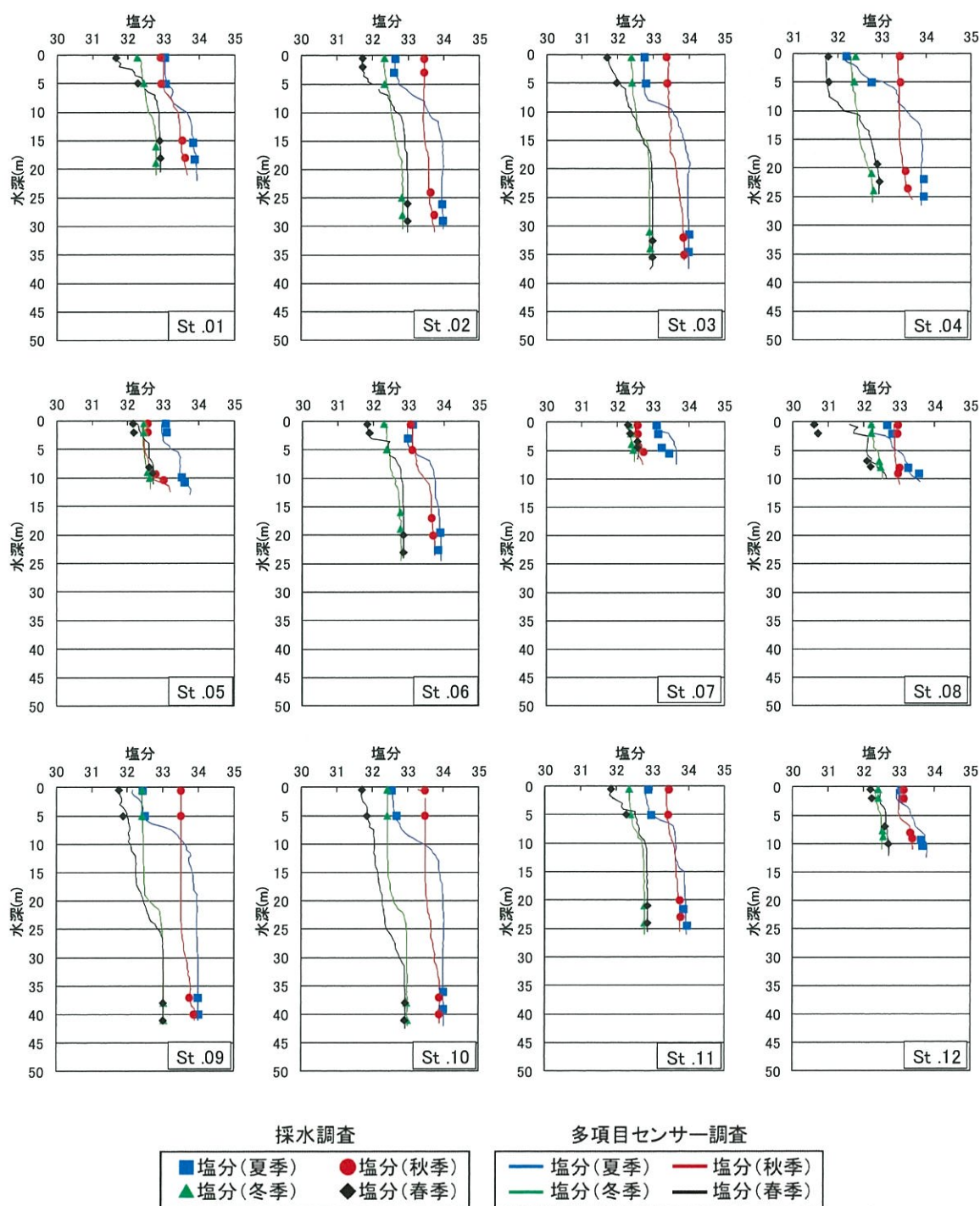
第 3.1-3 図 水質調査結果鉛直分布（塩分）
