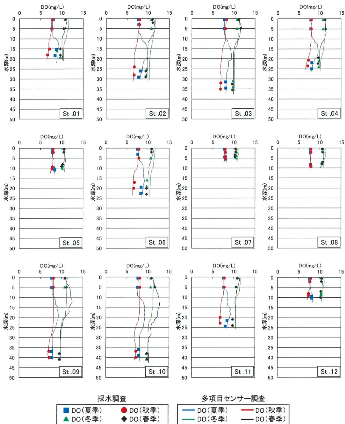
第 3.1-4 図 水質調査結果鉛直分布 (DO)
