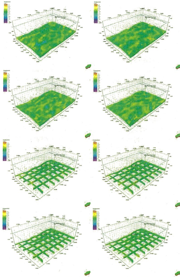
図 2.7-9 50 個の内 4 個の具現モデルの参考例：滝ノ上層 T 1 部層の孔隙率分布 (上図：全体表示、下図：格子状に断面を表示、図中の矢印は北を示す)
