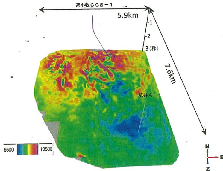
図 2.7-3 滝ノ上層 T1 部層下部の音響インピーダンス
