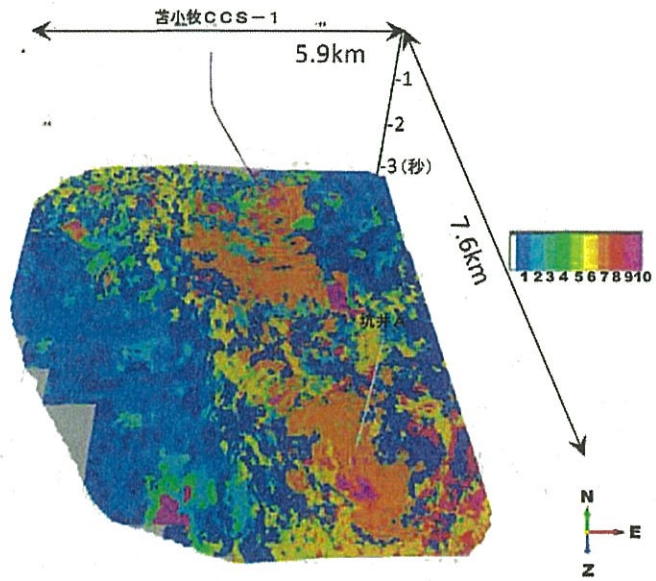
図 2.7-2 滝ノ上層 T1 部層下部の岩相分布 (K-means Index)
