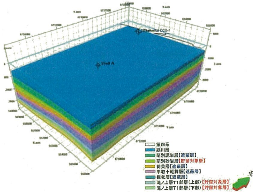
図 2.7-6 三次元地質モデル鳥瞰図
