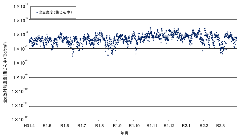
利尻測定所における大気浮遊じんの大α放射能濃度(集じん中)の経時変化
