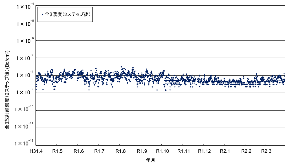
佐渡関岬測定所における大気浮遊じん全β放射能濃度(2ステップ後)の経時変化
