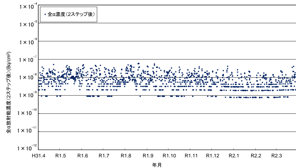
隠岐測定所における大気浮遊じん全α放射能濃度(2ステップ後)の経時変化
