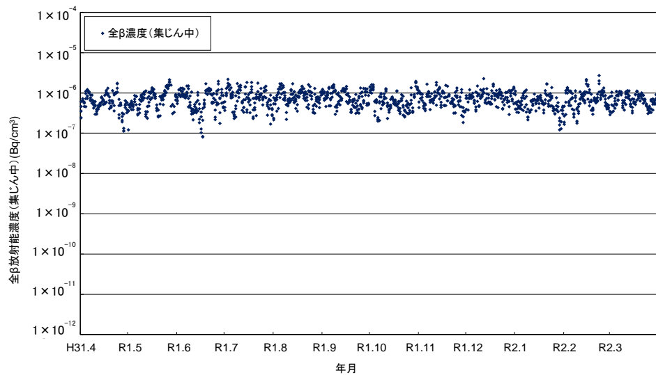
佐渡関岬測定所における大気浮遊じん全β放射能濃度(集じん中)の経時変化
