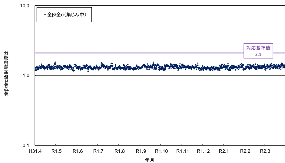
佐渡関岬測定所における大気浮遊じん全β/全α放射能濃度比(集じん中)の経時変化
